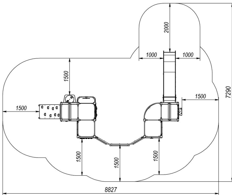
Рисунок 1 -Площа для монтажу та зона приземлення
