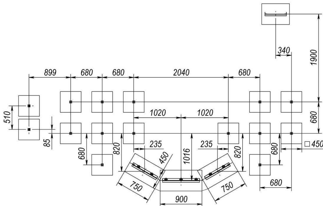
Рисунок 2 – Схема розташування фундаментів
