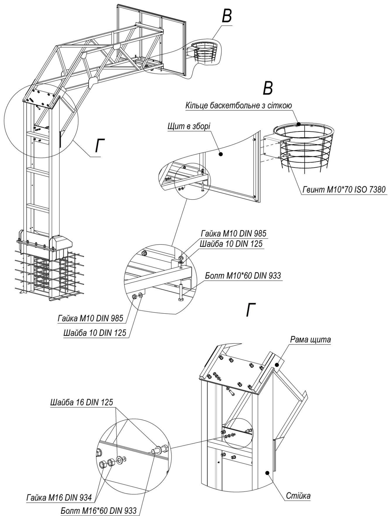
Рисунок 2 - Схема монтажу рами з щитом
