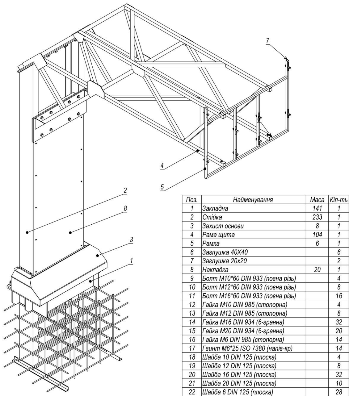
Рисунок 7 – УТ407.2
