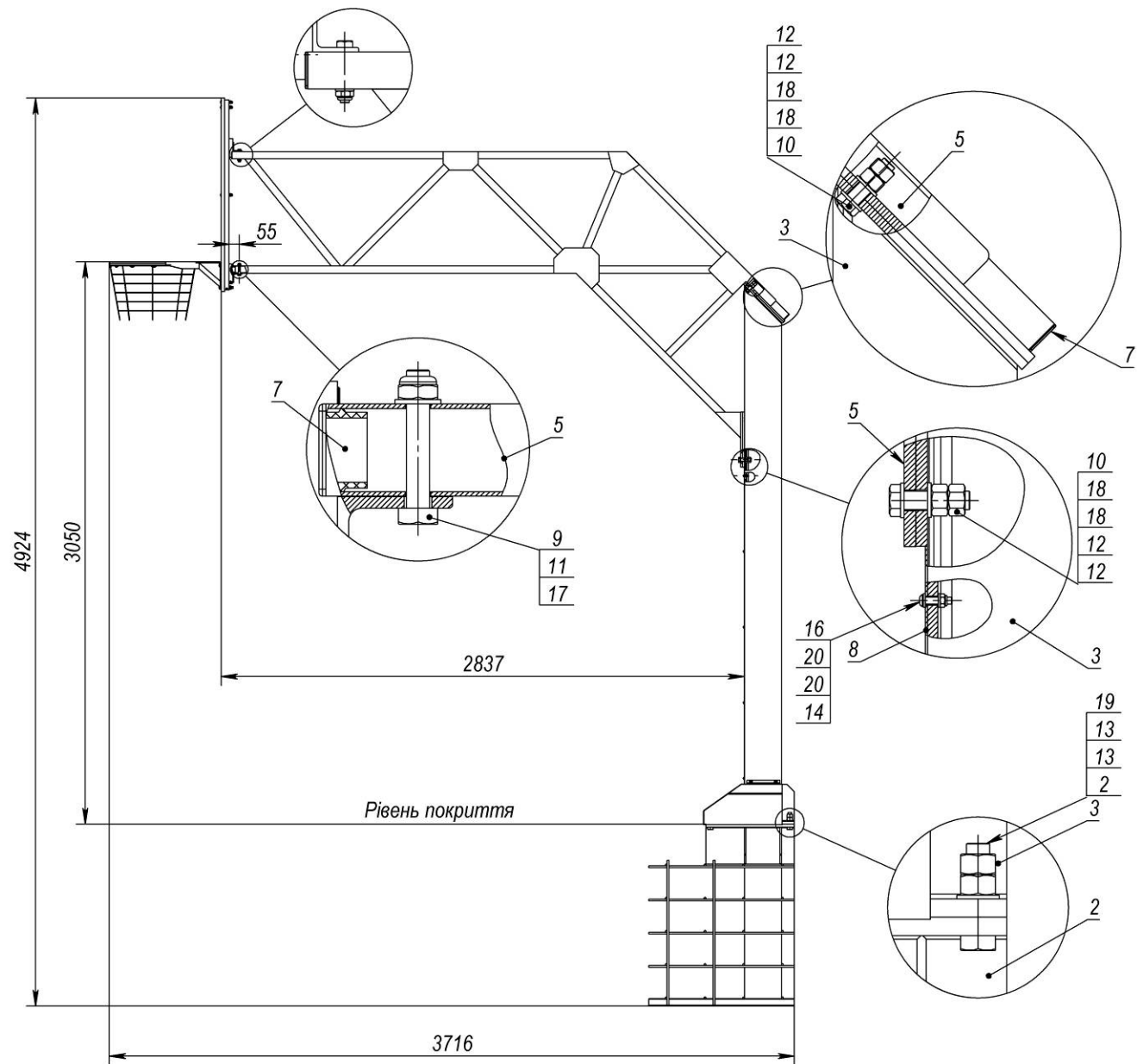
Рисунок 8 – УТ407.3
