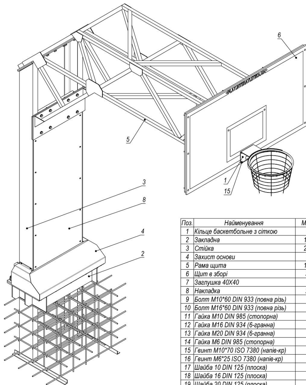
Рисунок 9 – УТ407.3
