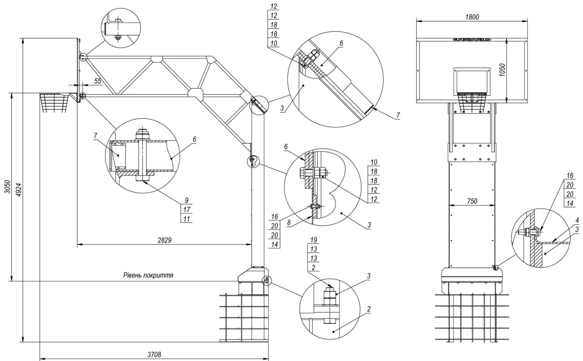
Рисунок 4 – УТ407.1
