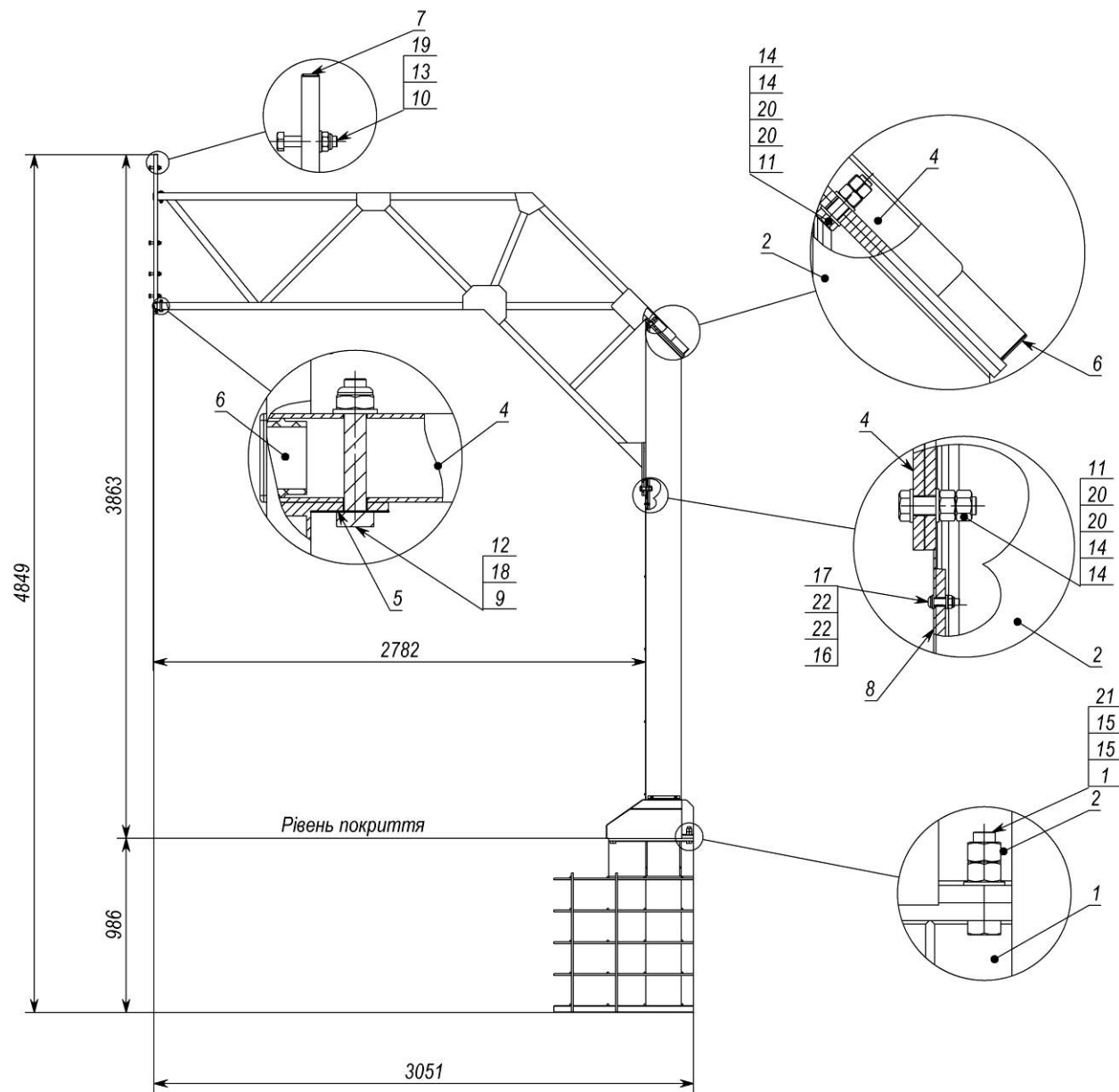
Рисунок 6 – УТ407.2
