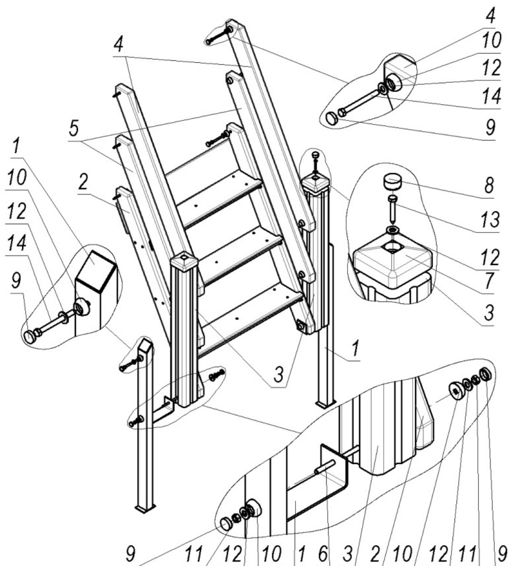
Рисунок 3 - Комплектність та схема складання даху
