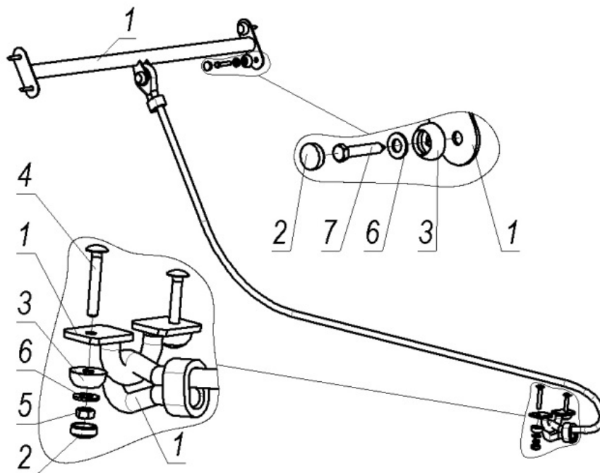
Рисунок 10 - Комплектність та схема кріплення стяжки
