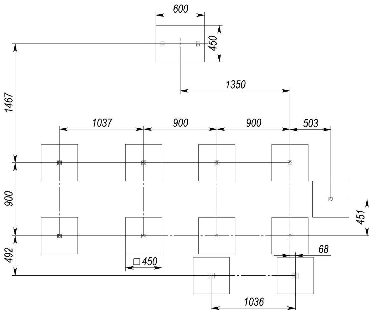
Рисунок 12 - Схема розташування фундаментів
