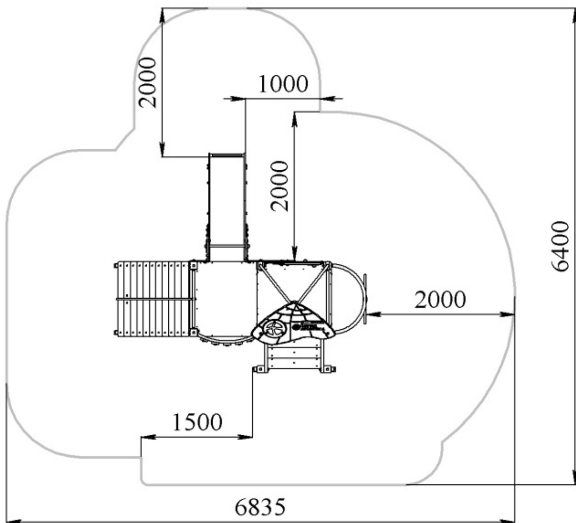
Рисунок 14 – Зона безпеки
