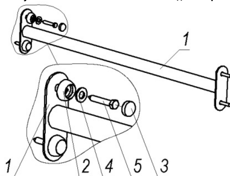
Рисунок 9 - Комплектність та схема складання гірки
