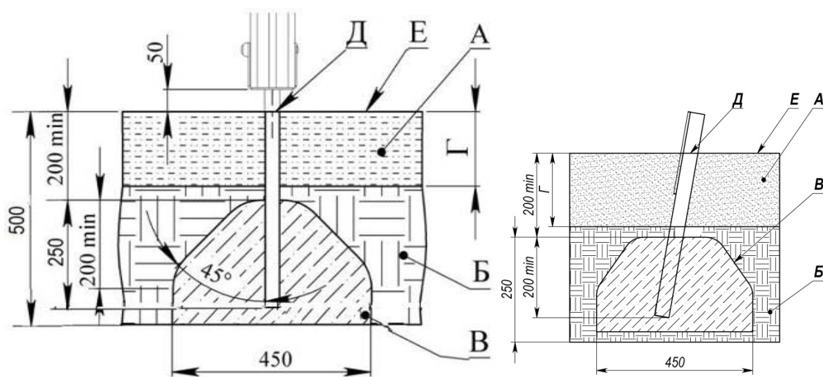
Рисунок 13 - Схема бетонування
