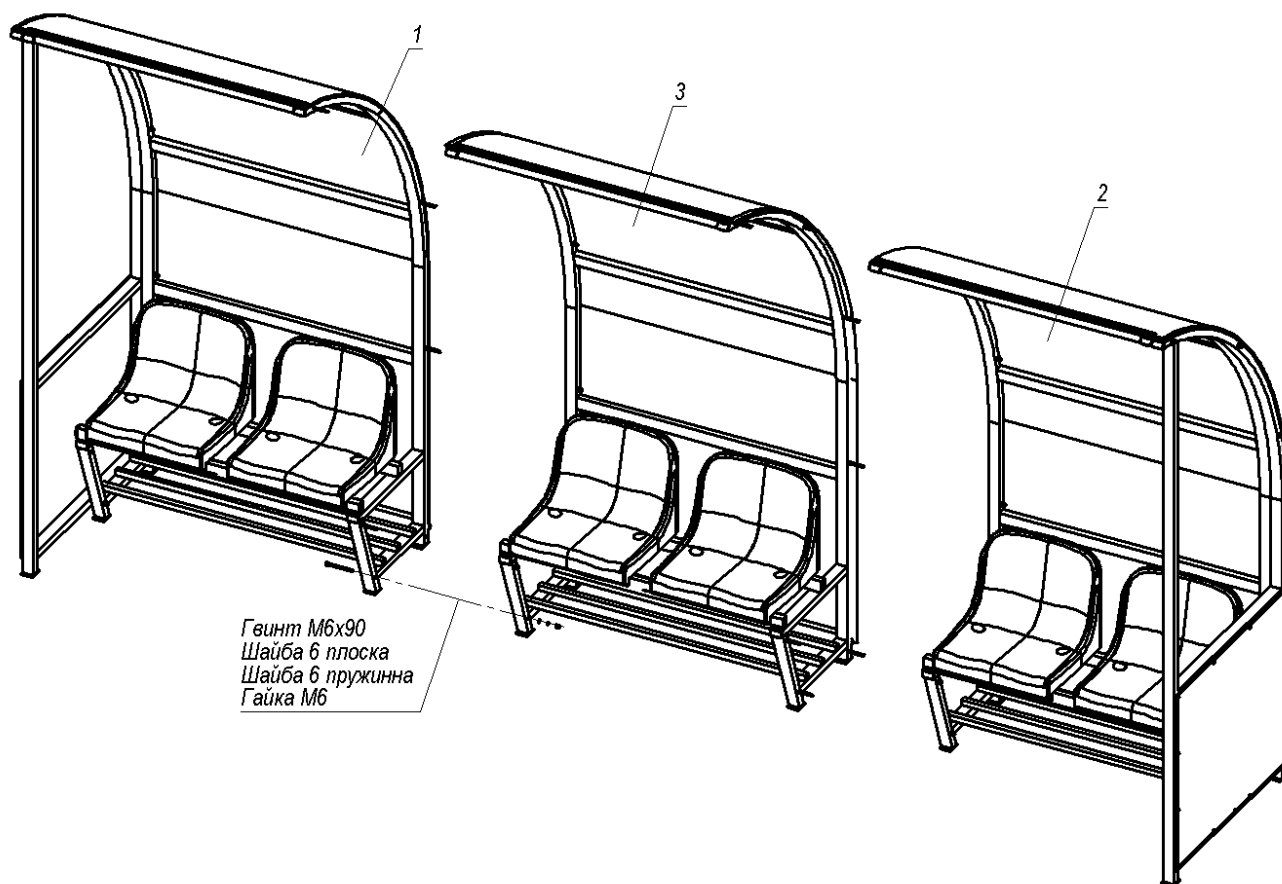
Рисунок 1 – Поділ виробу на складові частини
