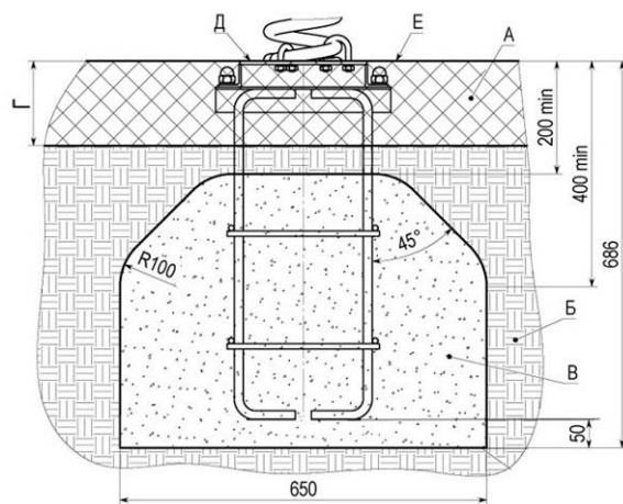
Рисунок 3 – Схема бетонування
