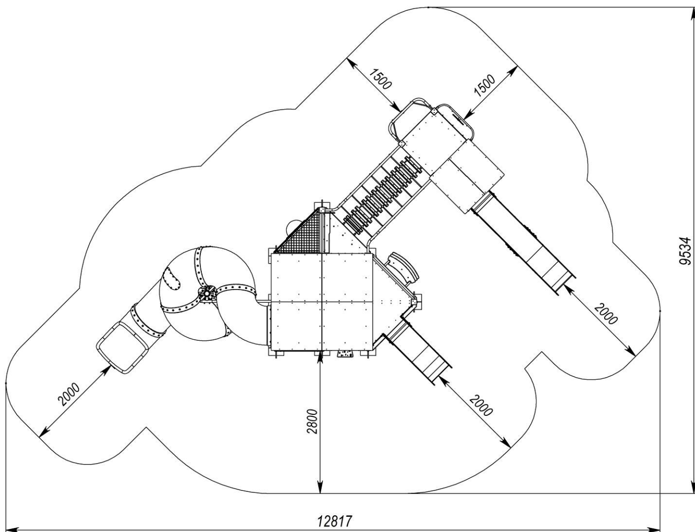
Рисунок 1 – Зона приземлення
