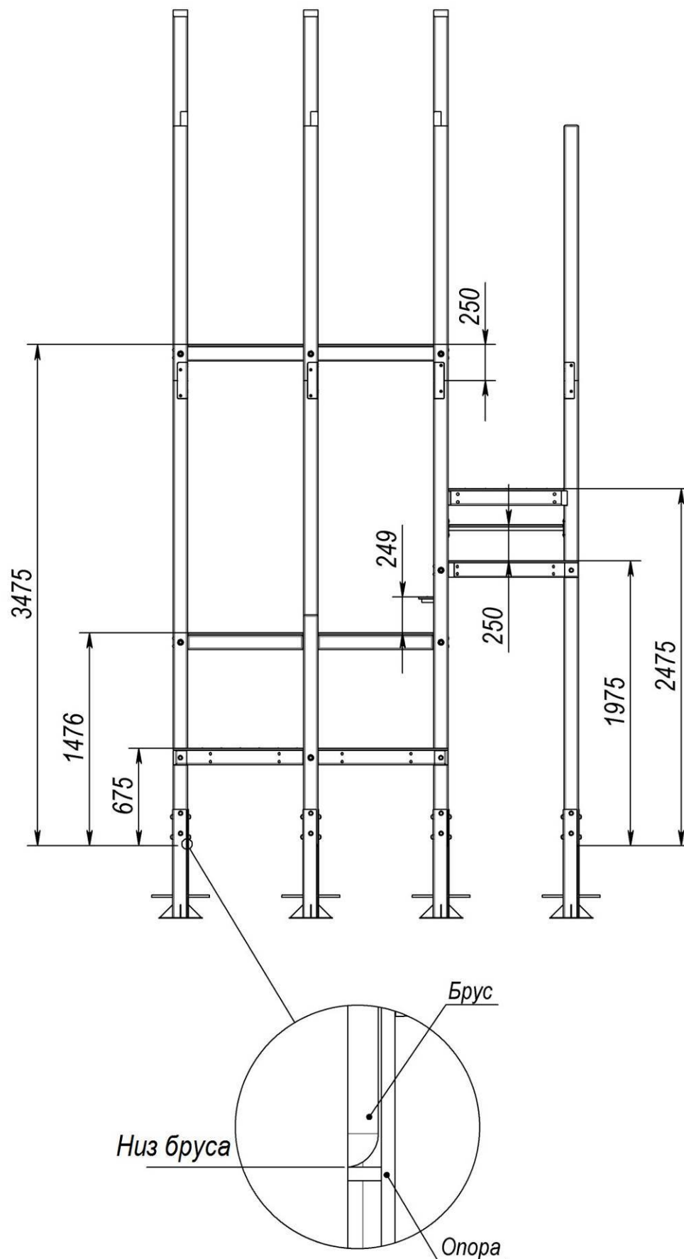
Рисунок 3 – Розташування площадок
