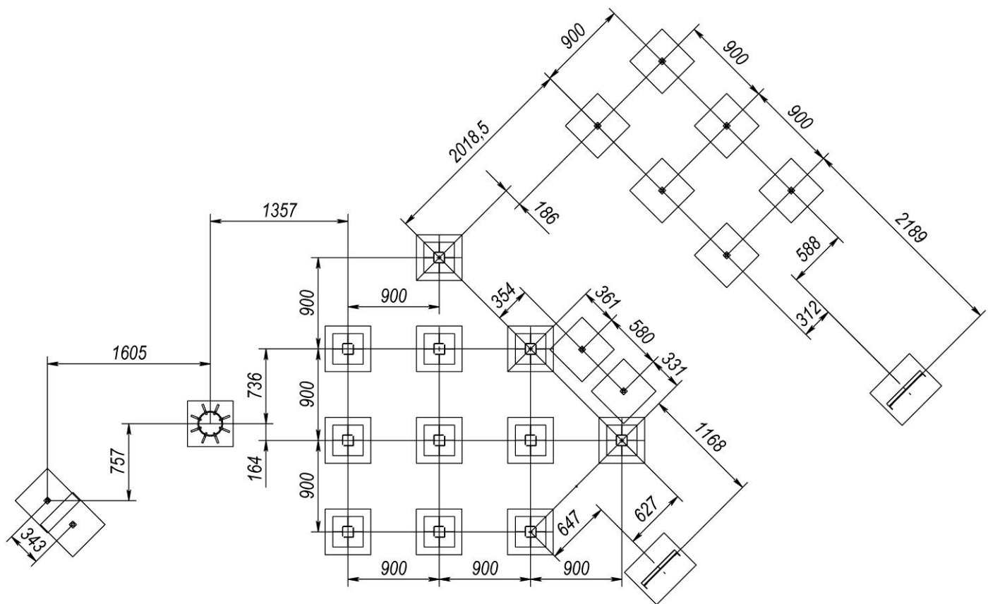
Рисунок 2 – Схема розташування фундаментів
