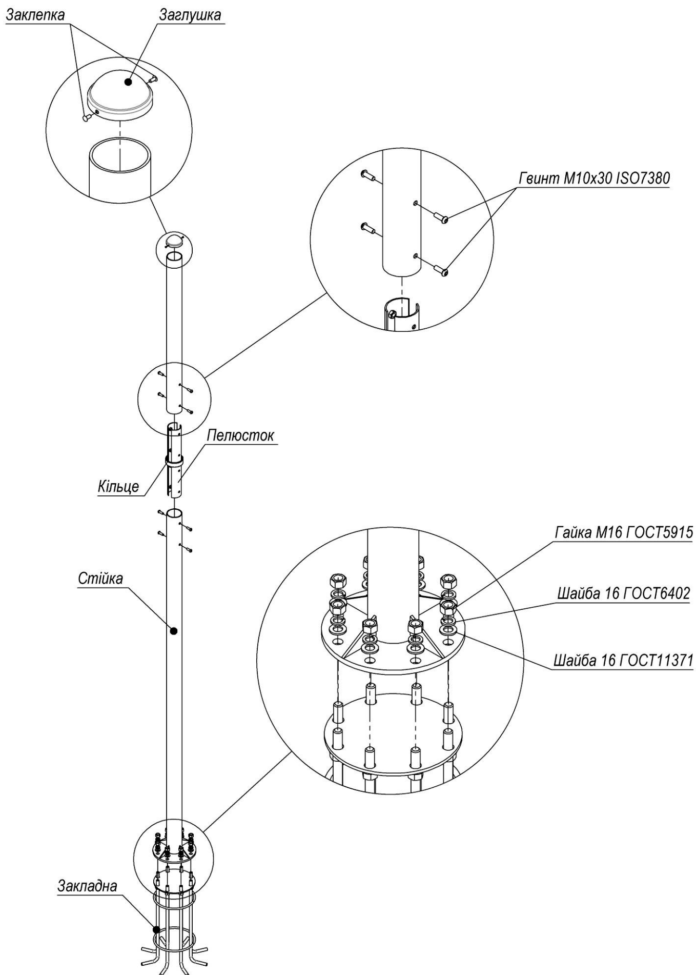
Рисунок 19 – Схема складання Стойки
