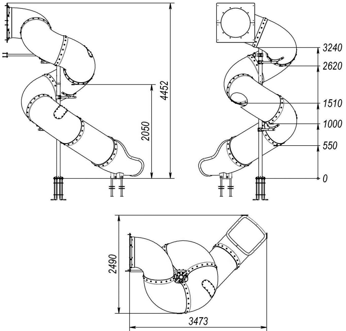
Рисунок 18 – Габаритні розміри
