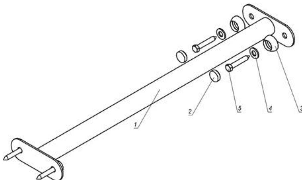
Мал. 6 - Комплектність та схема драбини дугової
