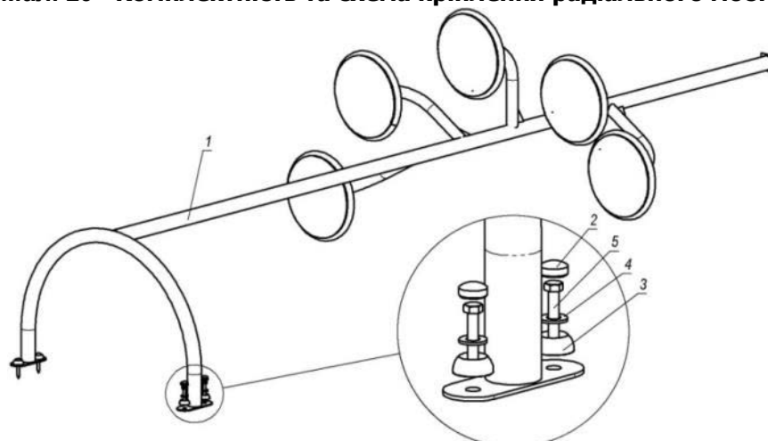
Мал. 10 - Комплектність та схема кріплення радіального моста
