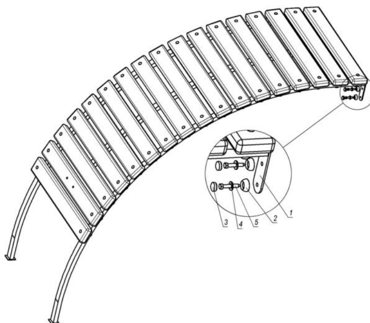
Мал. 11 – Схема кріплення гвинтової драбини до ігрового комплексу
