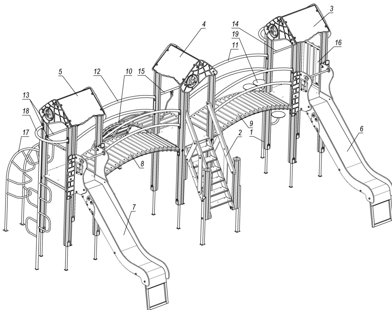
Мал. 1 - Комплектація та характеристики складових частин виробу
