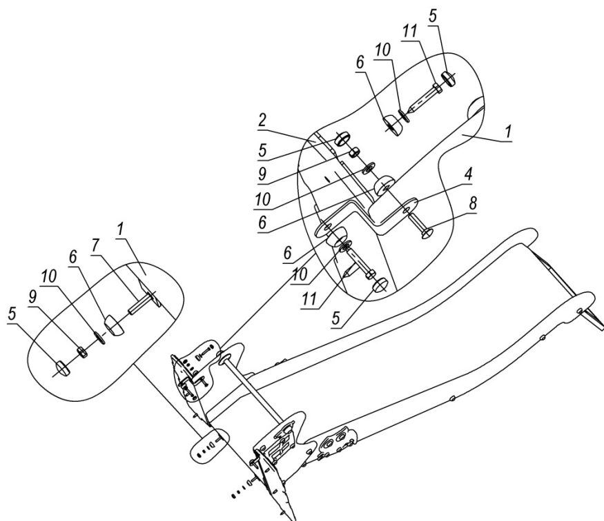
Мал. 7 - Комплектність та схема кріплення стяжки
