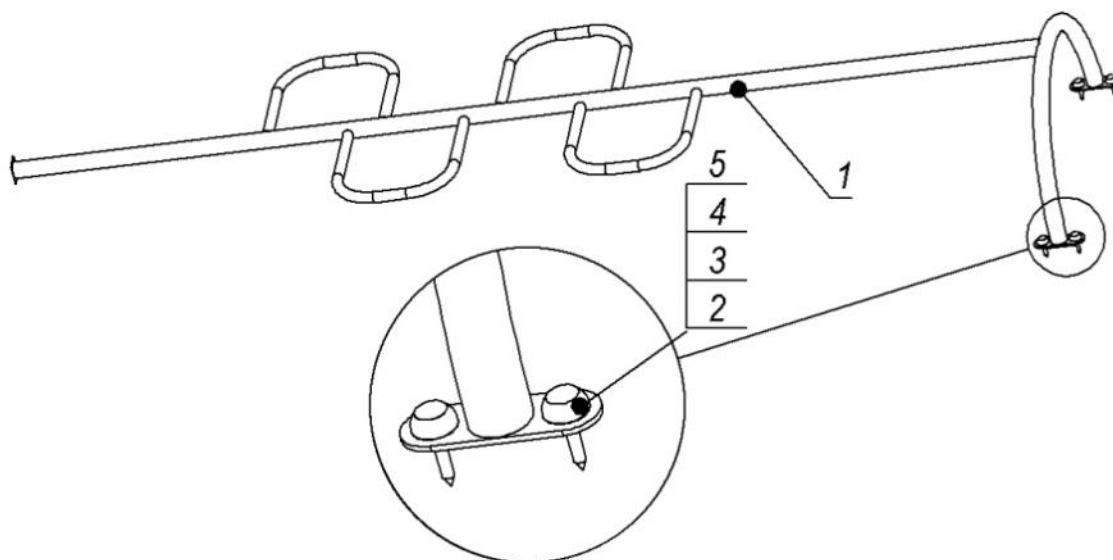
Мал. 5 - Комплектність та схема складання драбини дерев'яної
