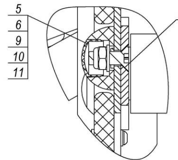
A-A (1 : 2)
