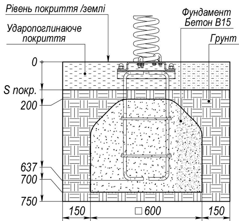
Рисунок 5 - Схема бетонування закладної (Поз. №3 в Додатку)
