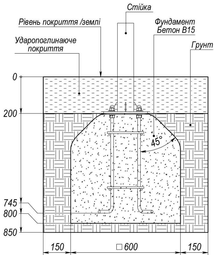
Рисунок 4 - Схема бетонування закладної (Поз. №5 в Додатку)
