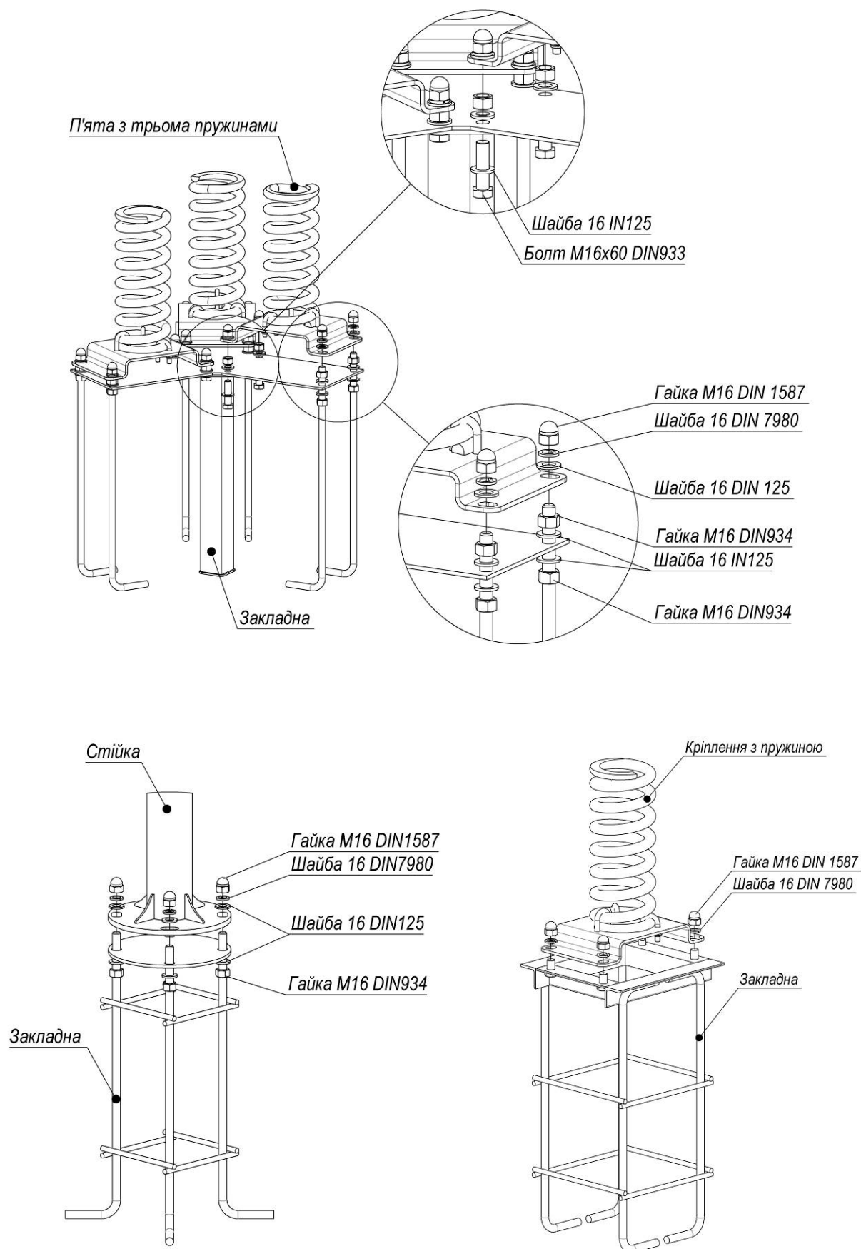
Рисунок 1 – Схема складання закладних
