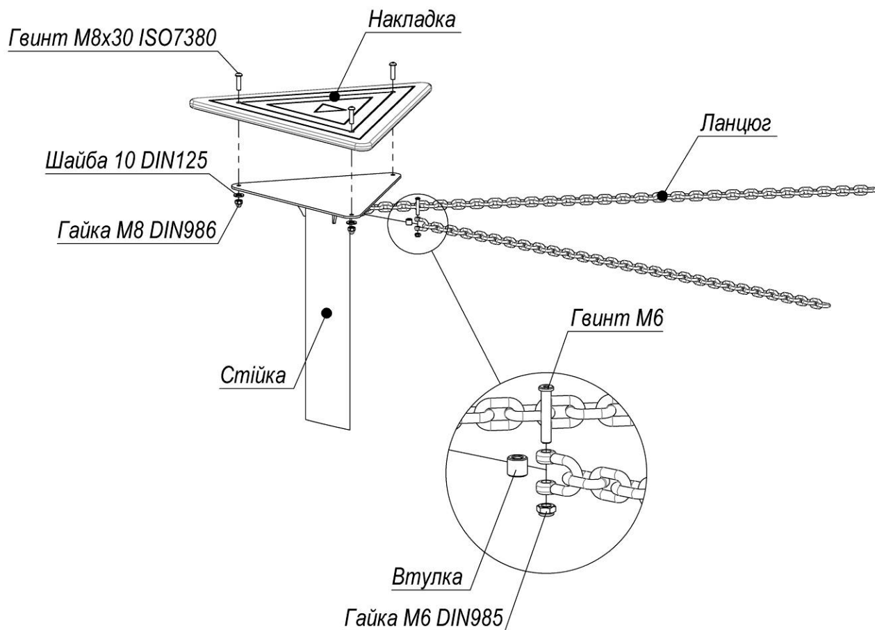
Рисунок 2 – Схема закріплення накладок та ланцюгів
