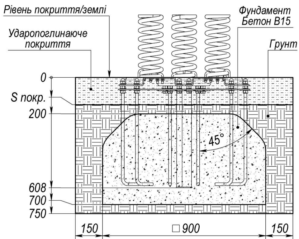
Рисунок 3 - Схема бетонування центральної закладної
