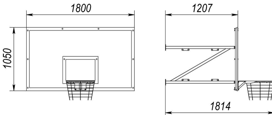
Рисунок 2 – Габаритні розміри для УТ409-1.2
