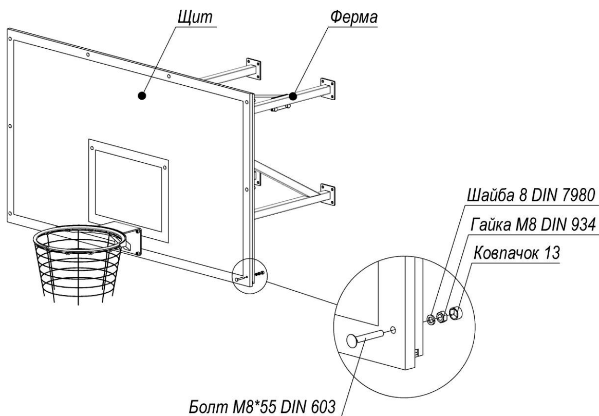
Рисунок 5 – Схема кріплення щита для УТ409-1.2
