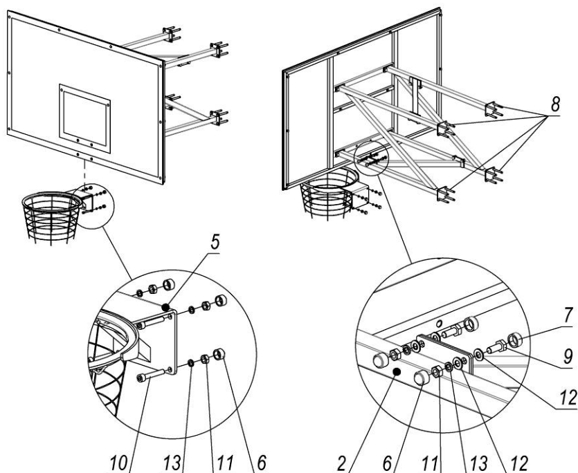
Рисунок 3 – Схема збирання 1
