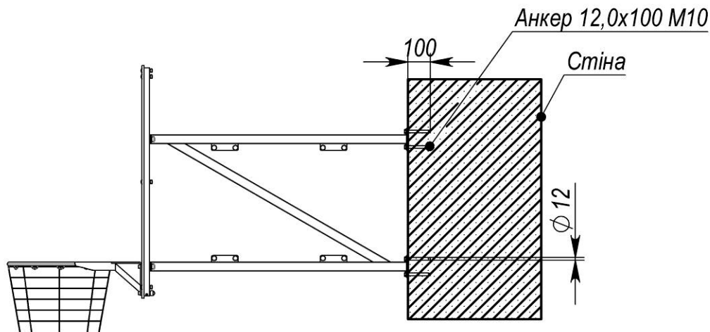
Рисунок 6 – Схема монтажу
