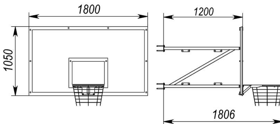
Рисунок 1 – Габаритні розміри для УТ409.1-1.2
