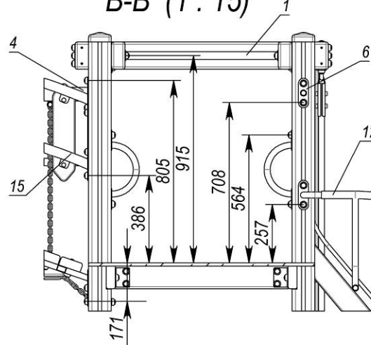
В-В (1 : 15)
