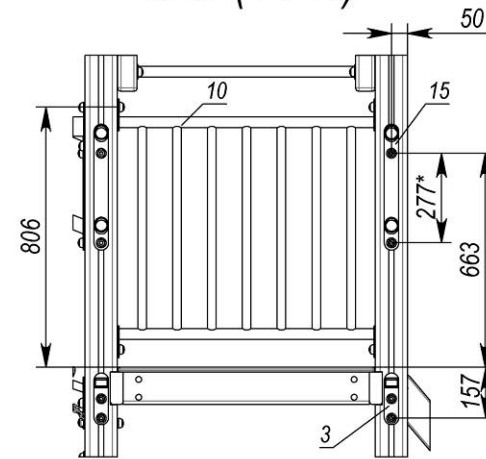
Б-Б (1 : 15)
