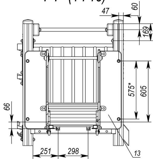
Г-Г (1 : 15)
