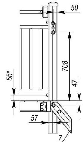
Д-Д (1 : 15)
