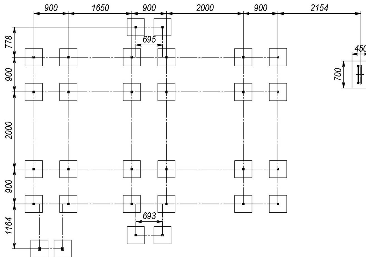
Схема розташування фундаменту
