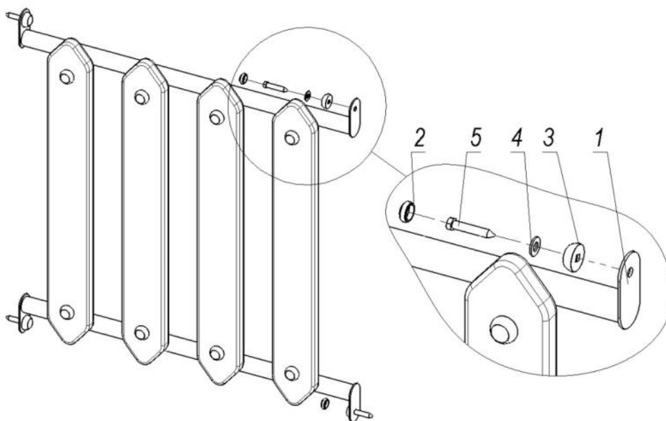
Рисунок 32 - Комплектність та схема складання перил Павук прямих
