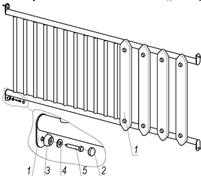
Рисунок 30 - Комплектність та схема складання перил мосту
