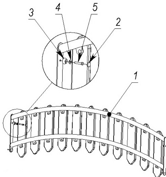
Рисунок 28 - Комплектність та схема складання огорожі в зборі
