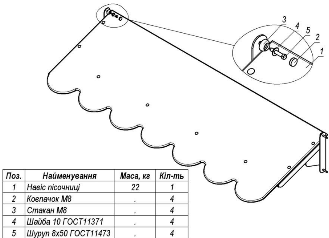
Рисунок 37 – Комплектація та схема кріплення навісу для пісочниці
