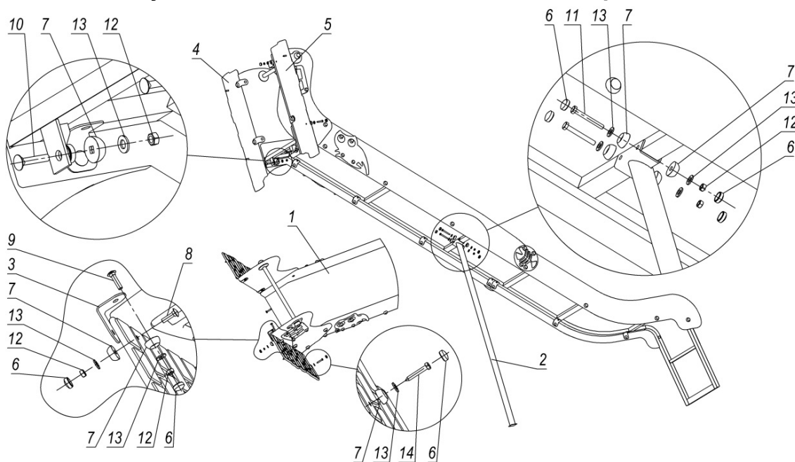
Рисунок 14 - Комплектність та схема складання гірки 0,7м
