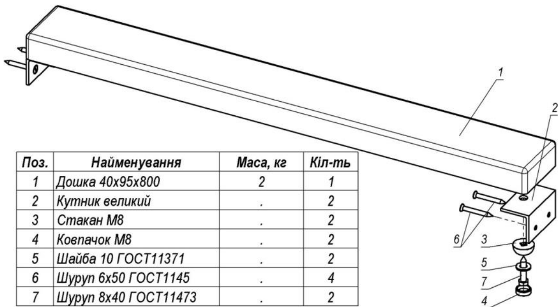
Рисунок 25 – Комплектність та схема кріплення переходу дерев'яного (між мостами)
