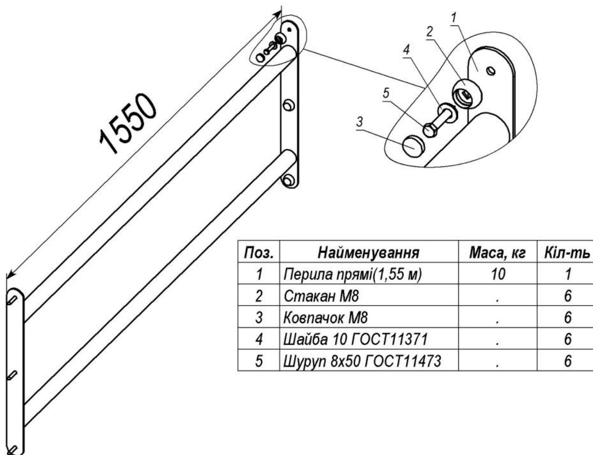
Рисунок 34 – Комплектність та схема кріплення перил прямих (1,55м)
