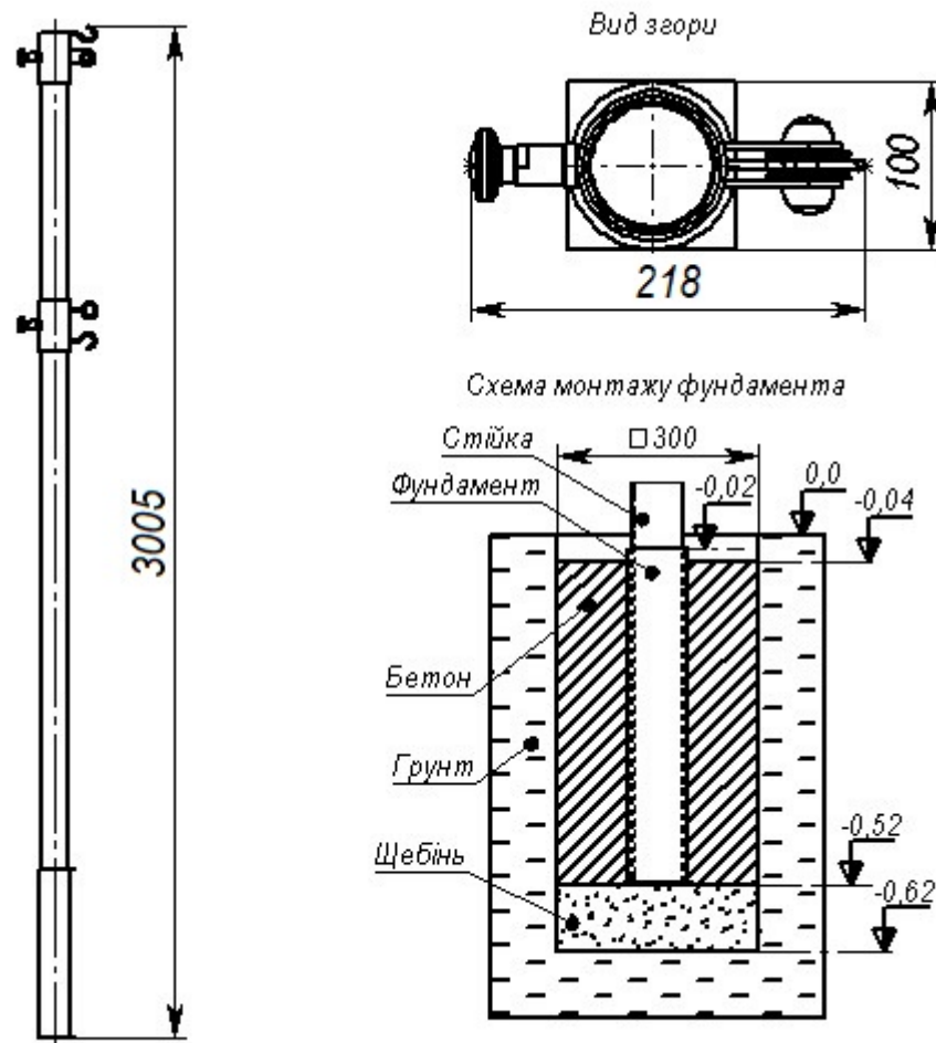
МАЛЮНОК 2 «Габаритні розміри виробу та схема монтажу»
