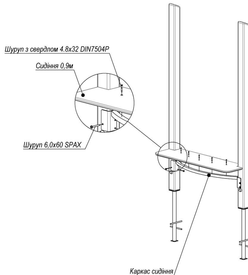
Рисунок 2 – Схема кріплення сидіння
