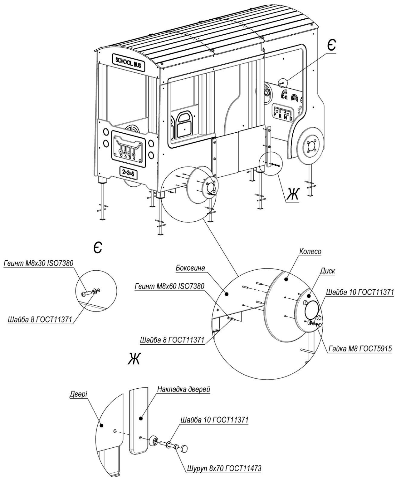
Рисунок 4 – Схема збирання коліс, накладок
