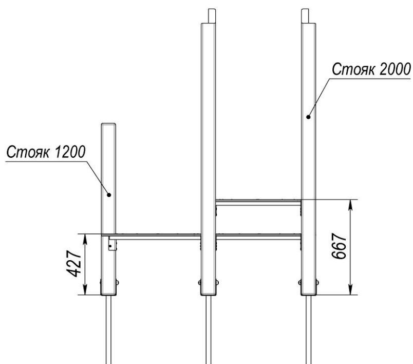
Рисунок 3 – Схема складання вежі
