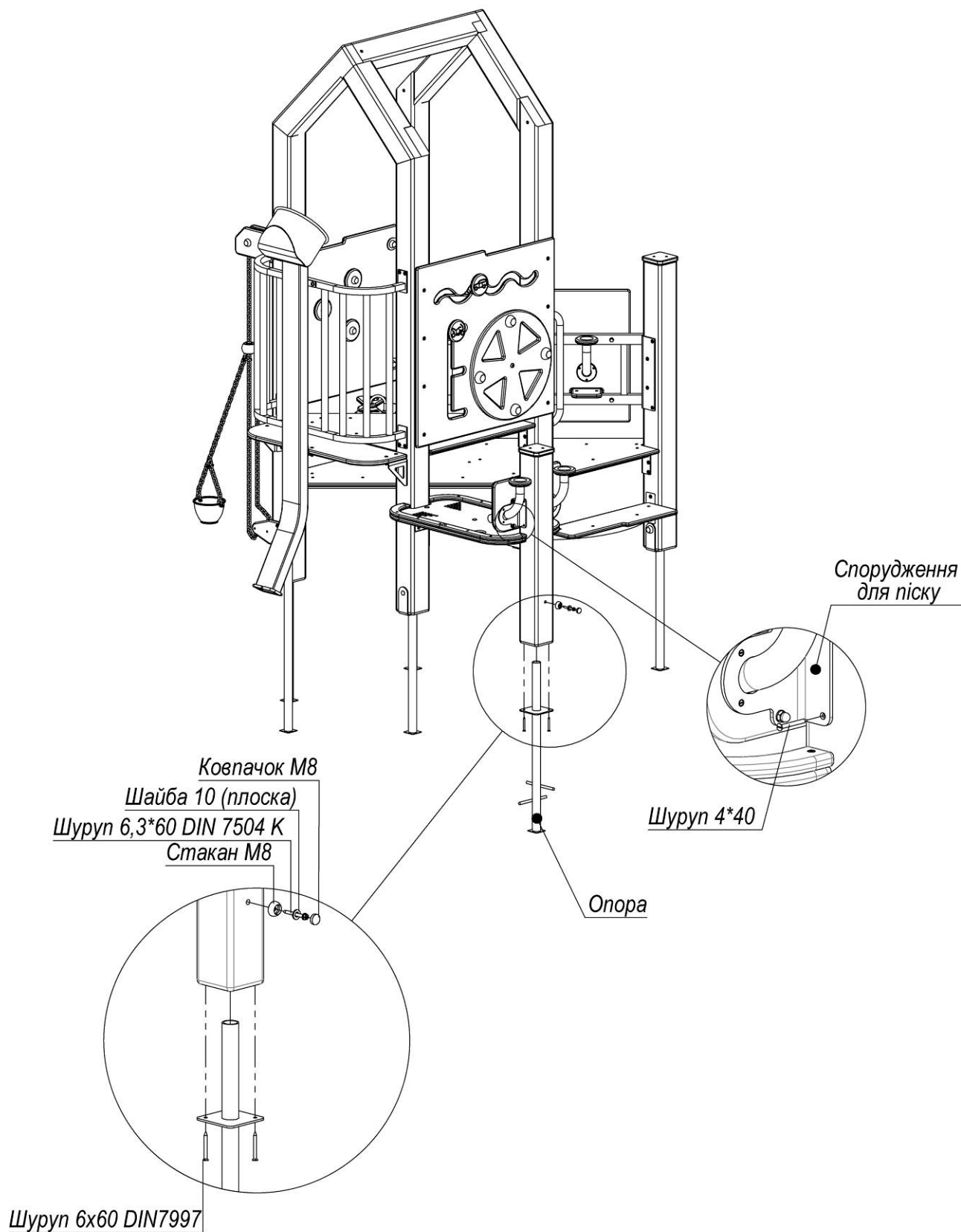
Рисунок 6 – Схема встановлення елементів комплексу
