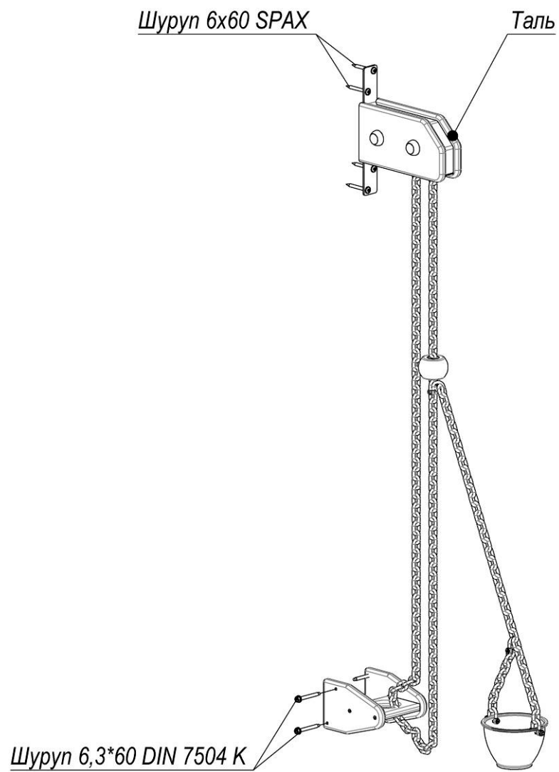
Рисунок 4 – Схема встановлення «Таль»
