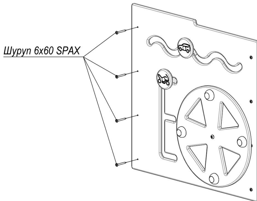
Рисунок 2 – Схема кріплення панелі (Кріплення інших панелей ідентичне)
