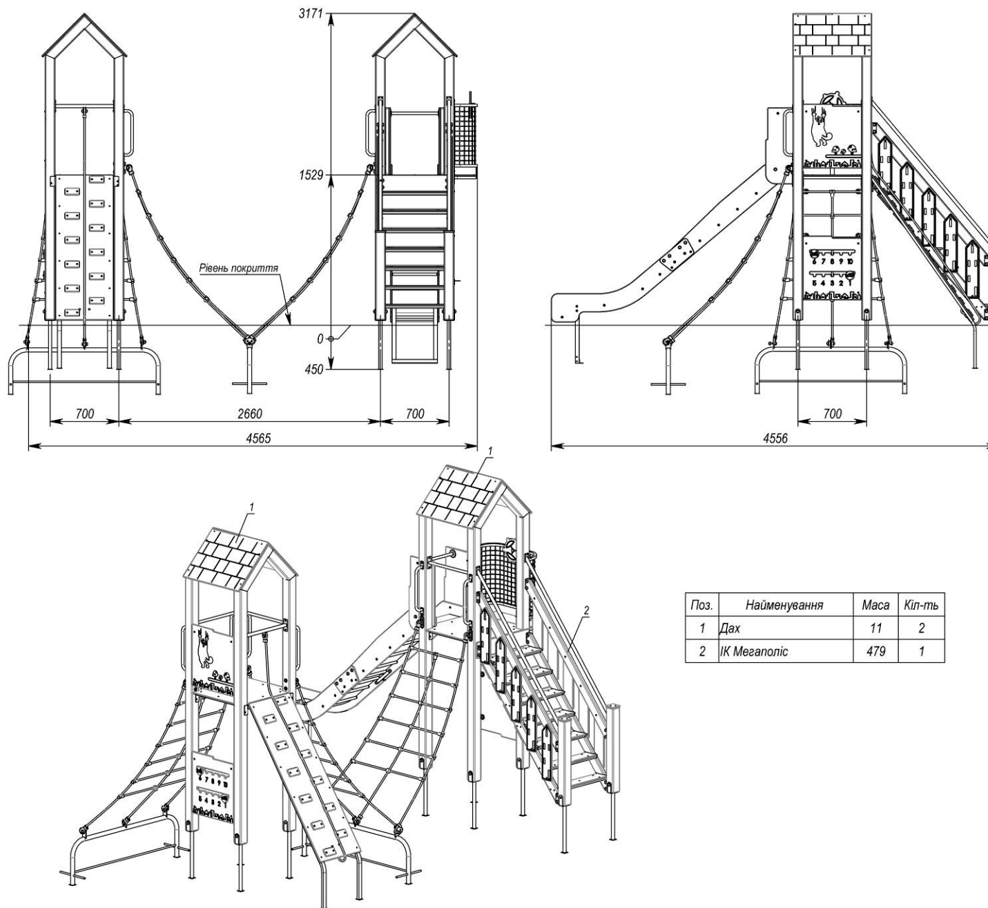
Рисунок 15 - Габаритні розміри комплексу для TE833(-PE)
