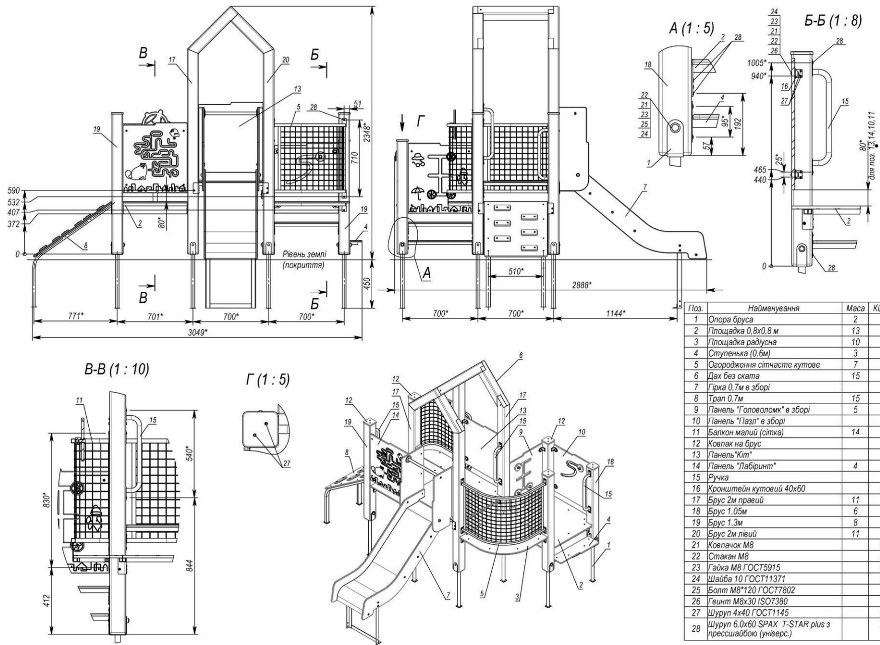
Рисунок 9 - Габаритні розміри комплексу для TE831-Base, -PE-Base
