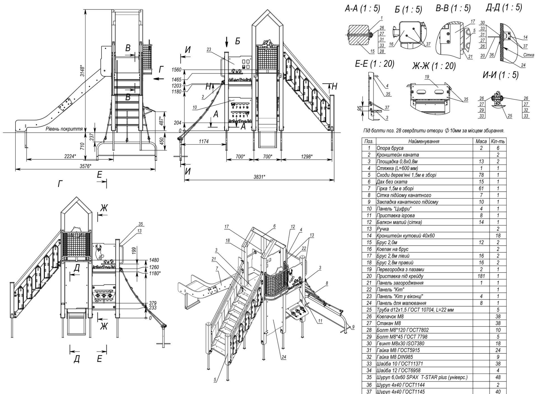
Рисунок 11 - Габаритні розміри комплексу для TE832-Base, -PE-Base
