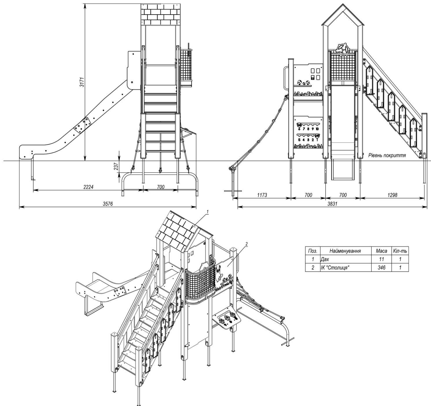
Рисунок 13 - Габаритні розміри комплексу для TE832(-PE)
