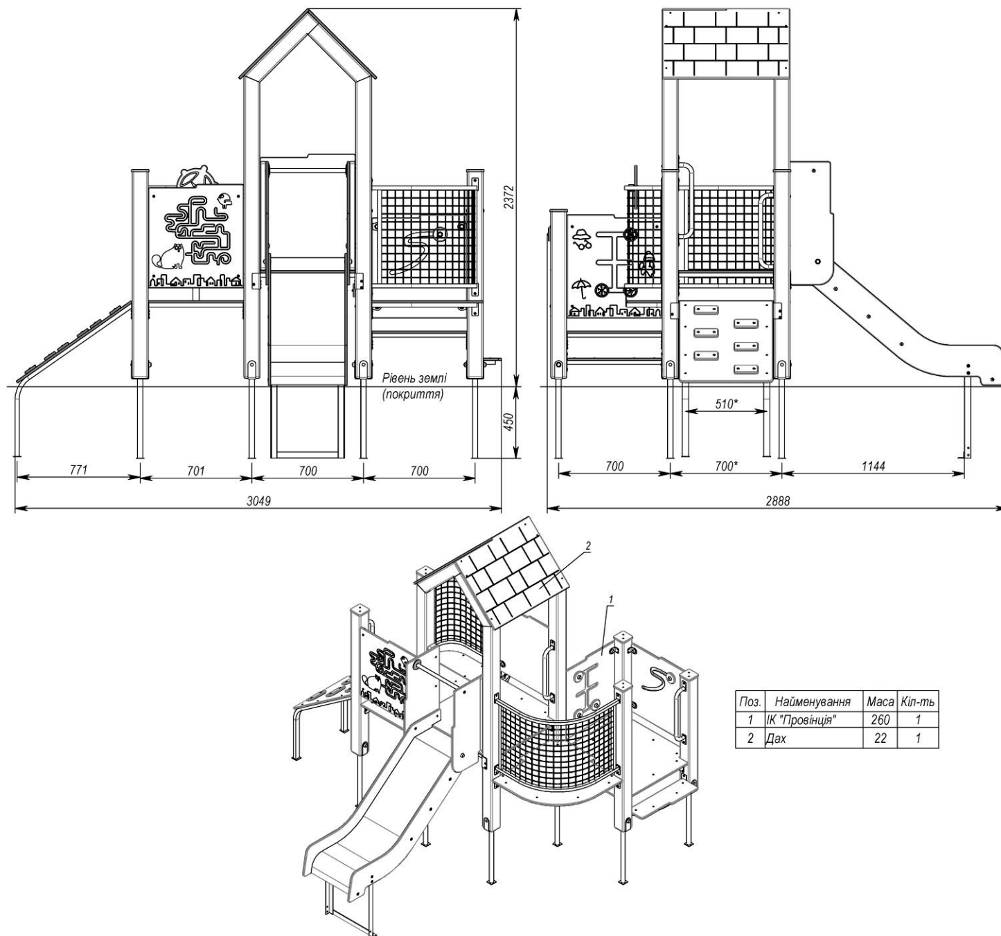
Рисунок 10 - Габаритні розміри комплексу для TE831(-PE)
