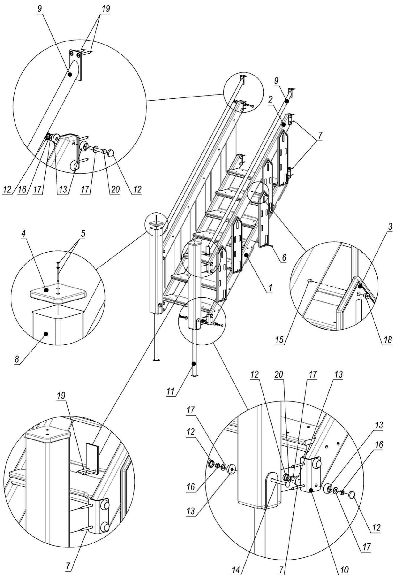
Рисунок 7 - Схема складання сходів для TE832, TE833
