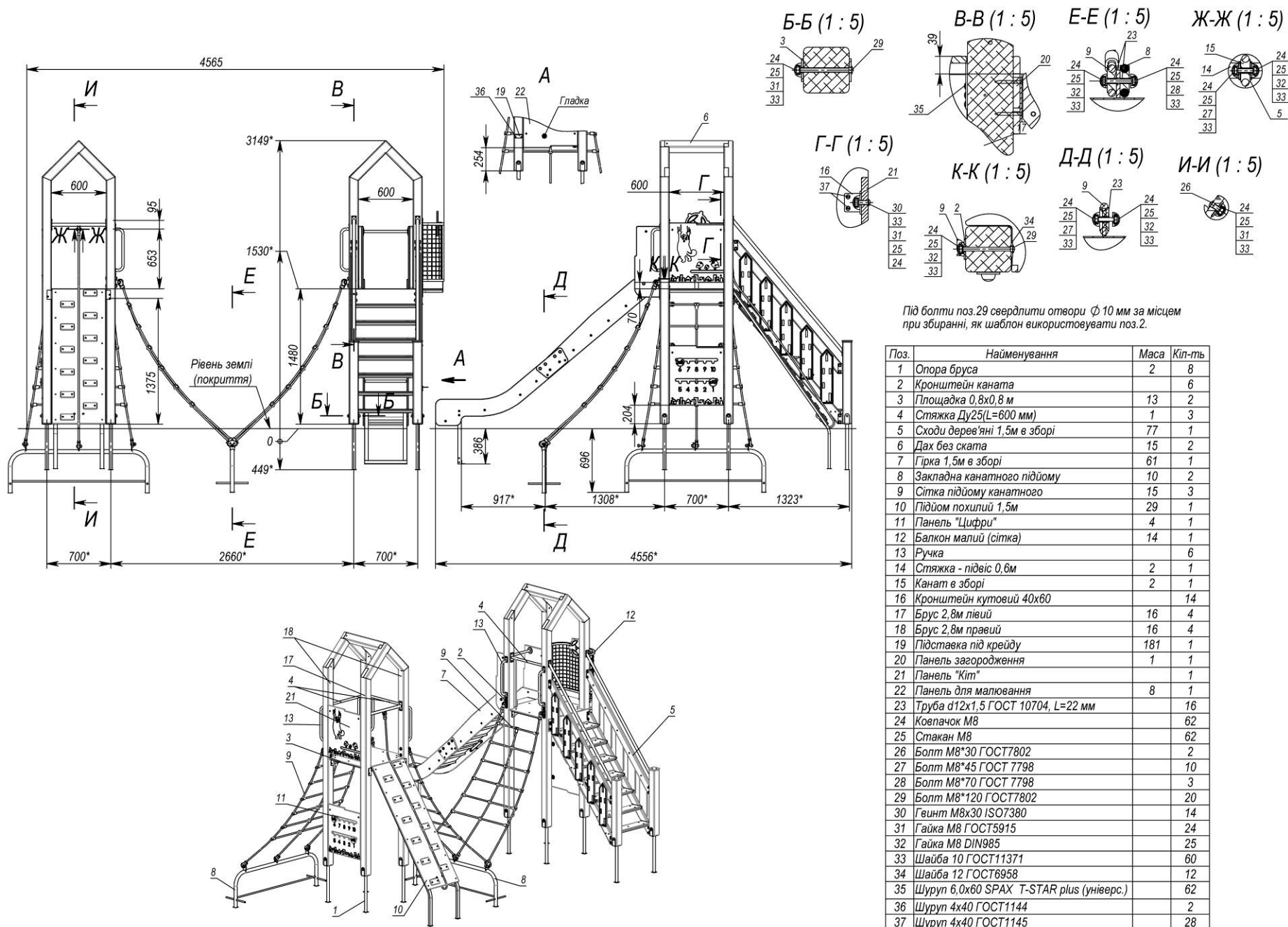
Рисунок 14 - Габаритні розміри комплексу для TE833-Base, -PE-Base
