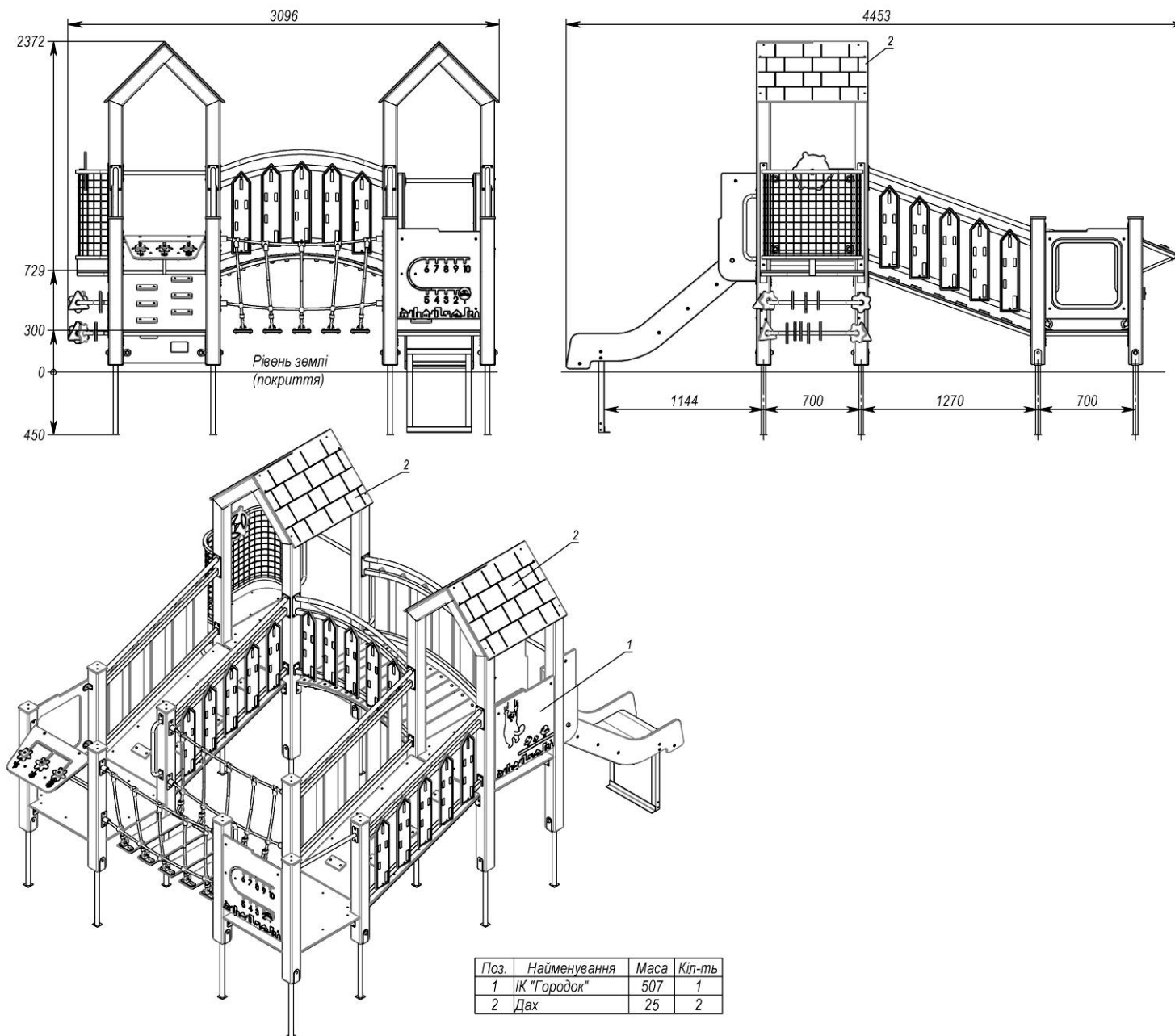
Рисунок 18 - Габаритні розміри комплексу для ТЕ834(-РЕ)
