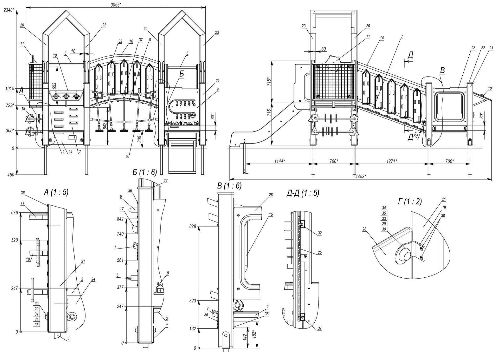
Рисунок 16 - Габаритні розміри комплексу для TE834-Base, -PE-Base
