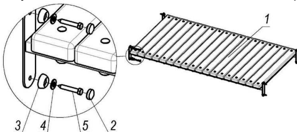
Рисунок 17 - Комплектність та схема складання ланцюгового мосту
