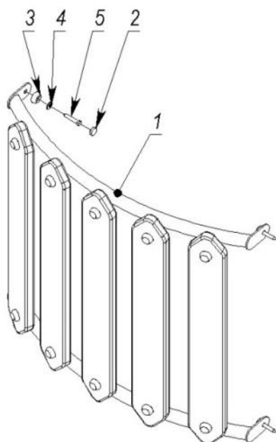
Рисунок 9 - Комплектність та схема складання гірки
