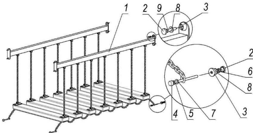
Рисунок 16 - Комплектність та схема складання сходів ступінчатих
