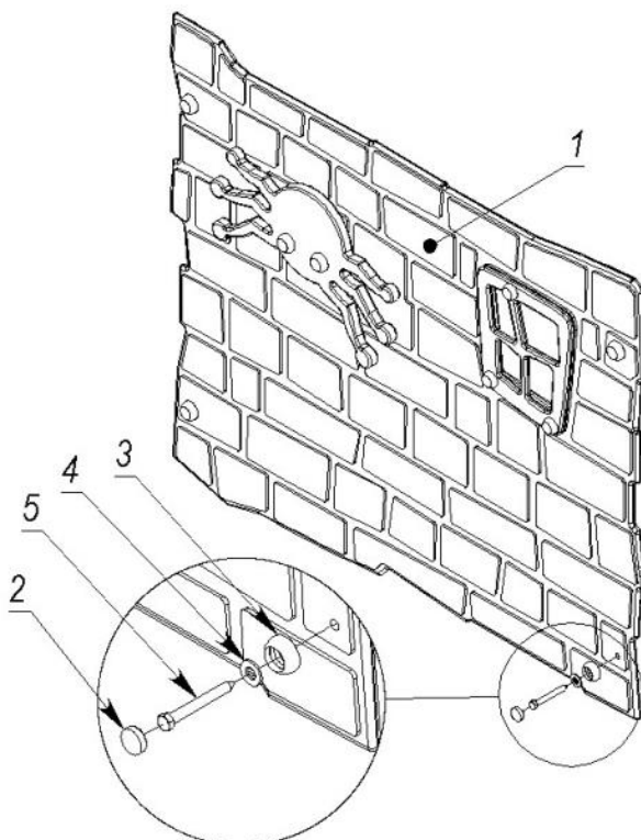
рисунок 7 - Комплектність та схема складання підйому
