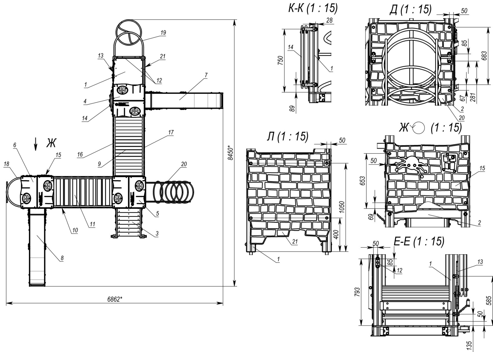
Рисунок 1 - Комплектація та характеристики складових частин виробу
