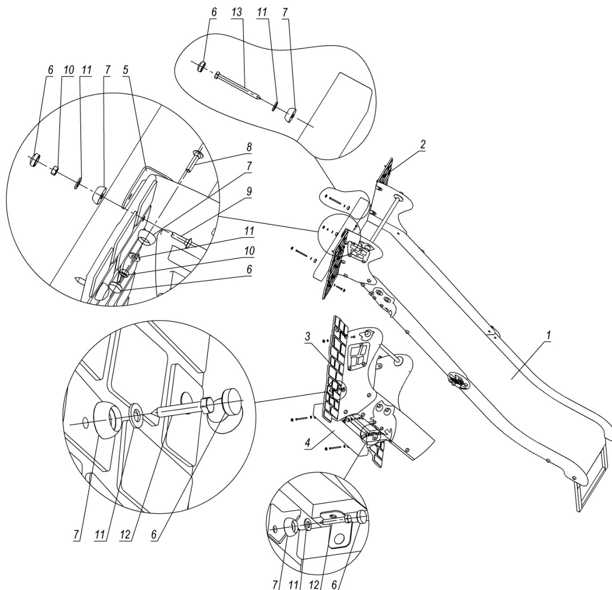
Рисунок 8 - Комплектність та схема складання панелі
