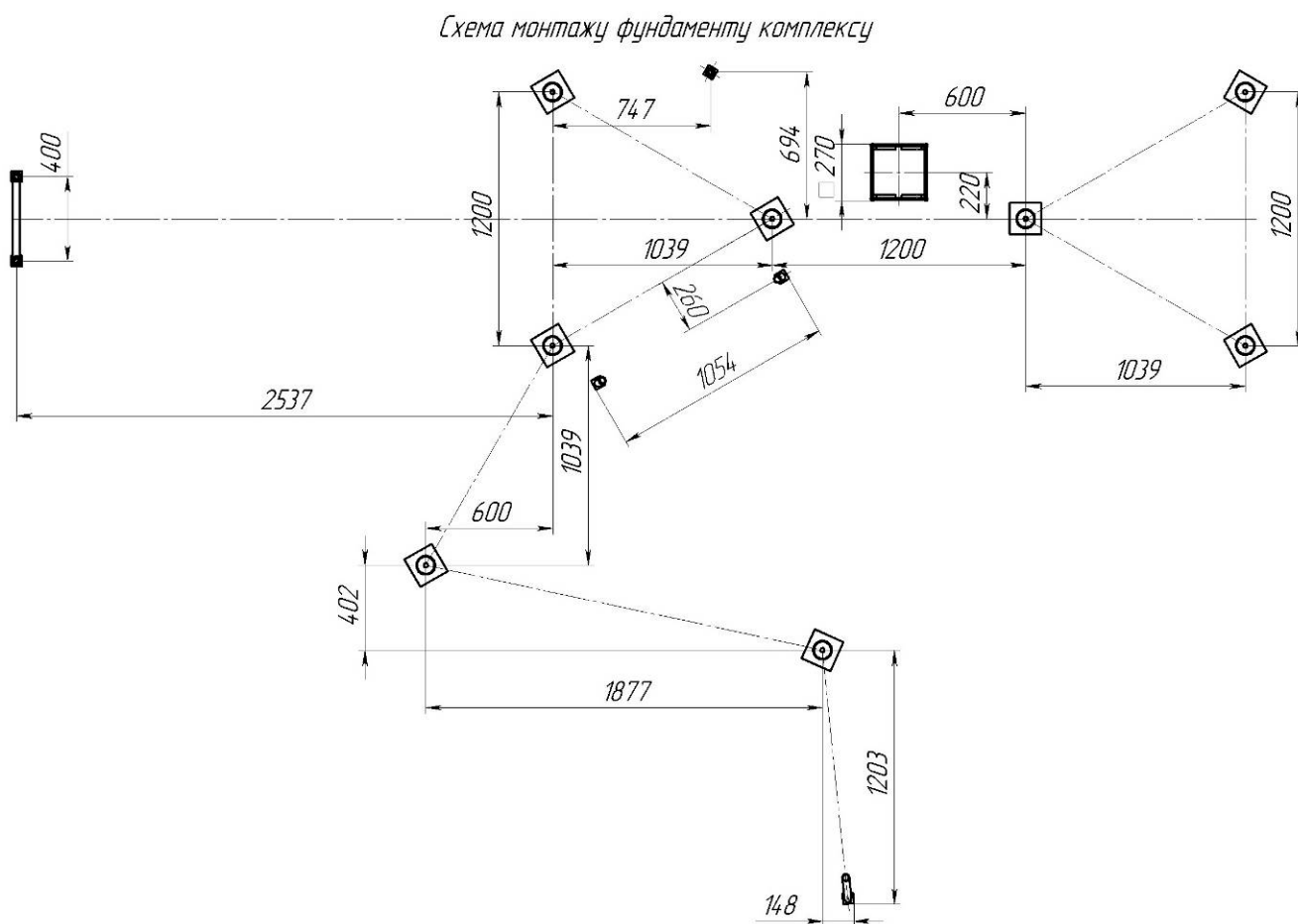
Мал. 8 - Схема розташування фундаментів
