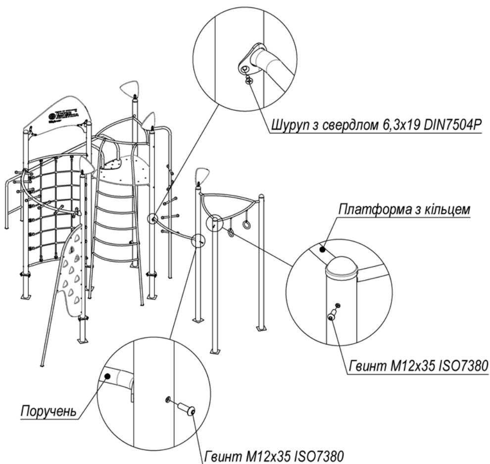
Мал. 6 - Комплектність та схема збірки поручня, платформи та кілець гімнастичних
