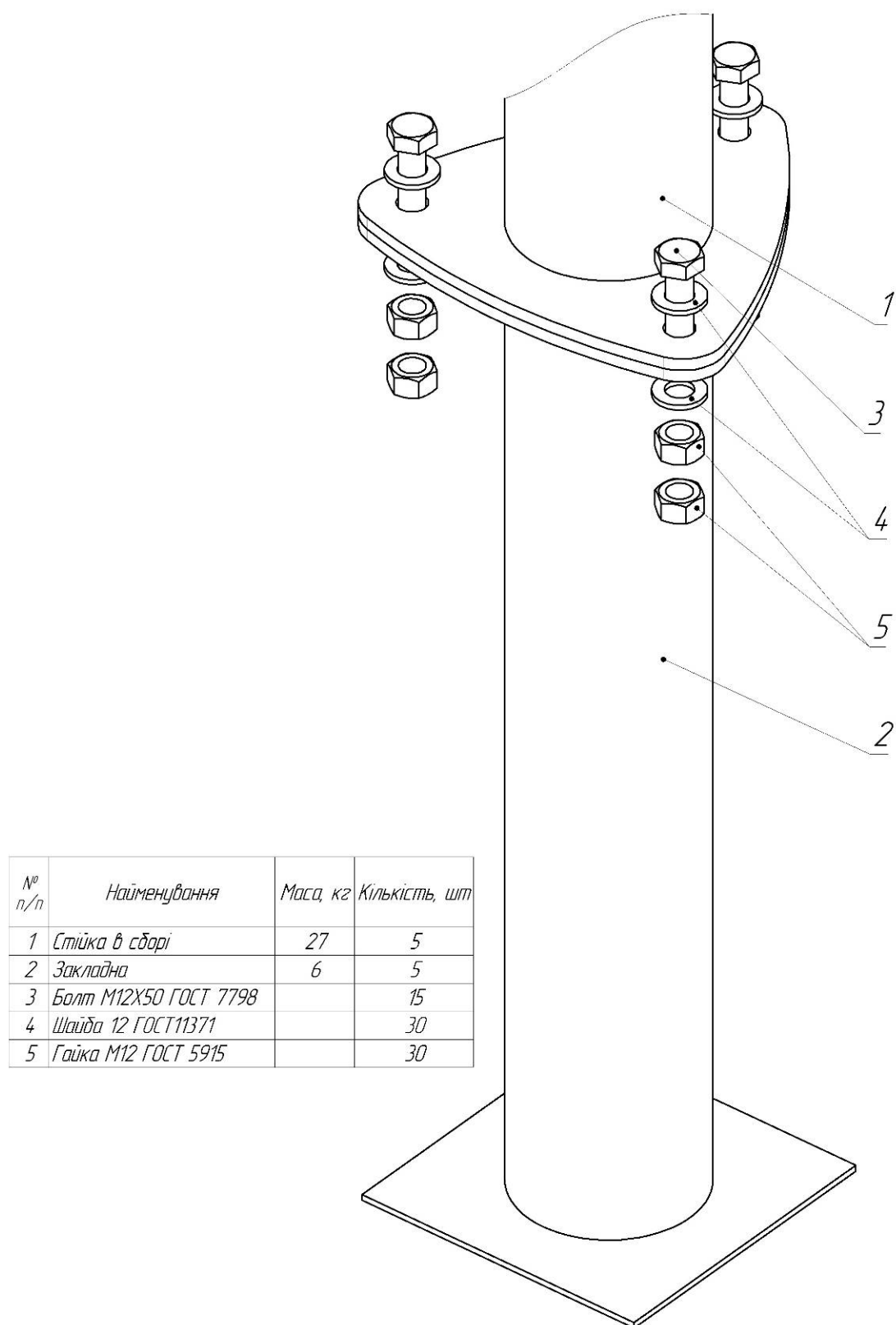
Мал. 1 - Комплектність та схема збірки стійок із закладною
