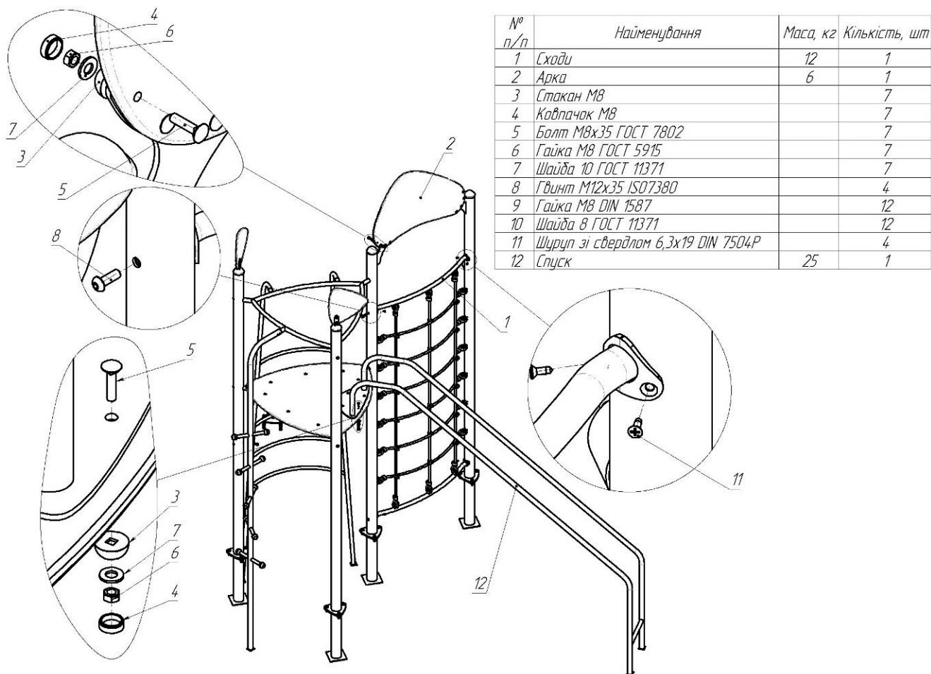
Мал. 4 - Комплектність та схема збірки сходів, арки та спуск
