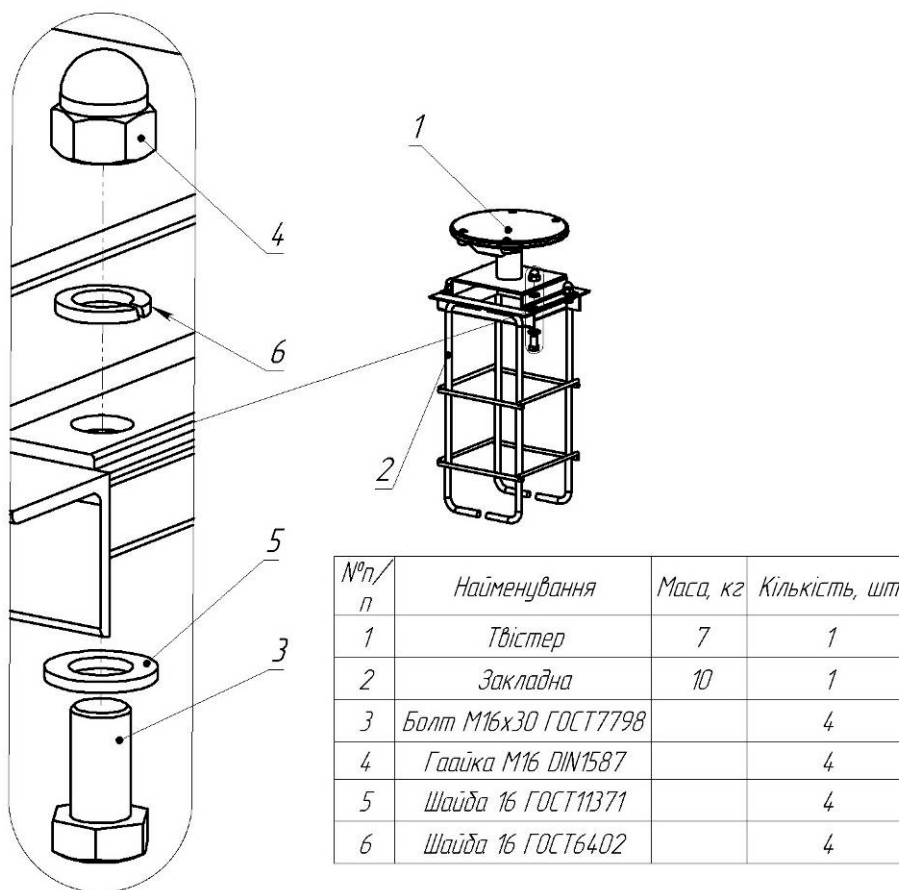
Мал. 7 - Комплектність та схема збірки твістеру
