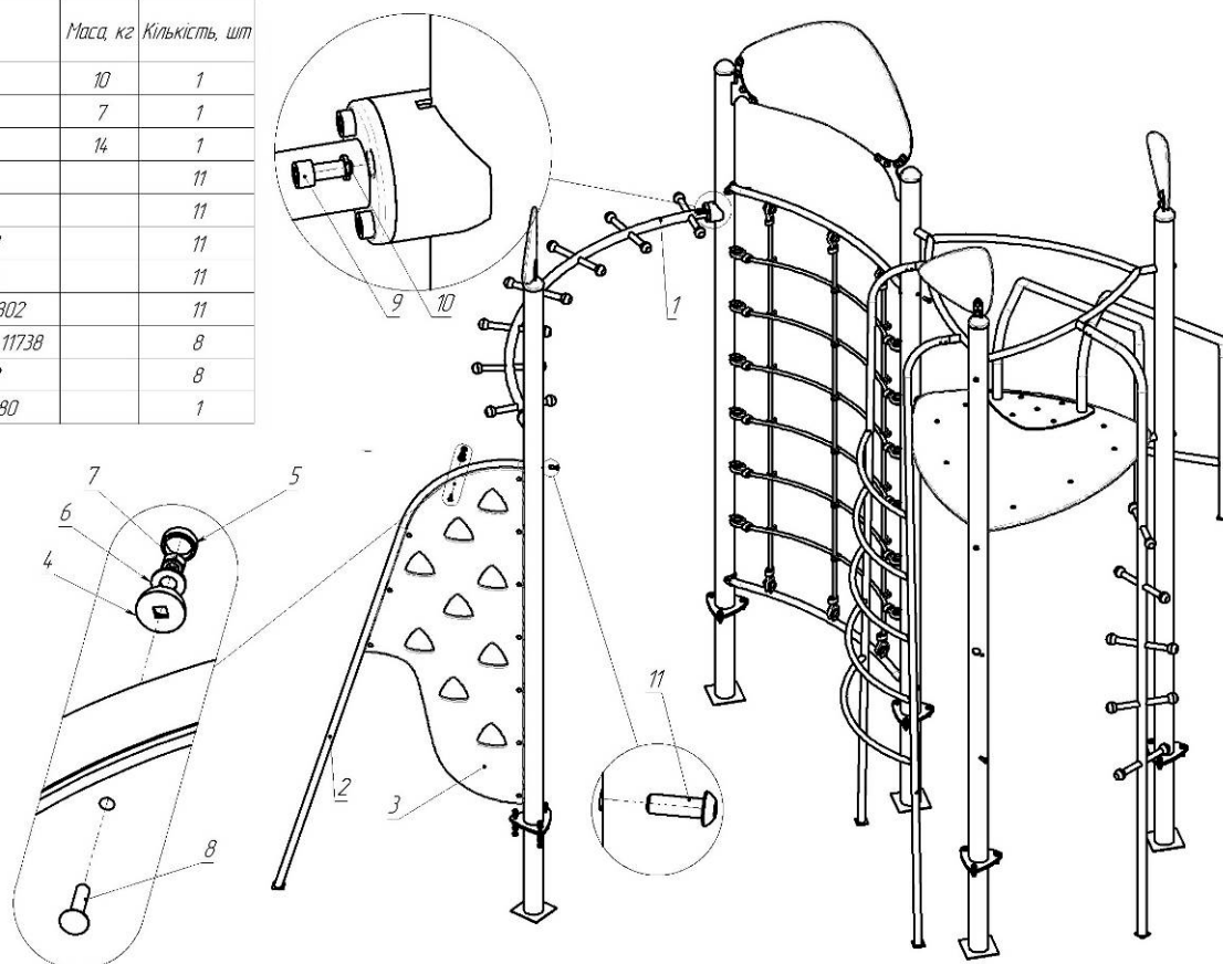
Мал. 5 - Комплектність та схема збірки руко ходу, стійки та підйому
