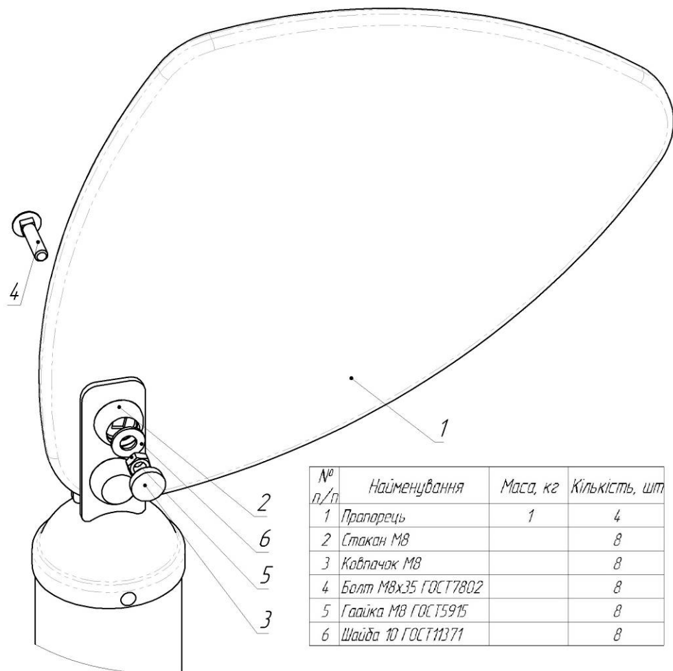
Мал. 3 - Комплектність та схема збірки прапорців
