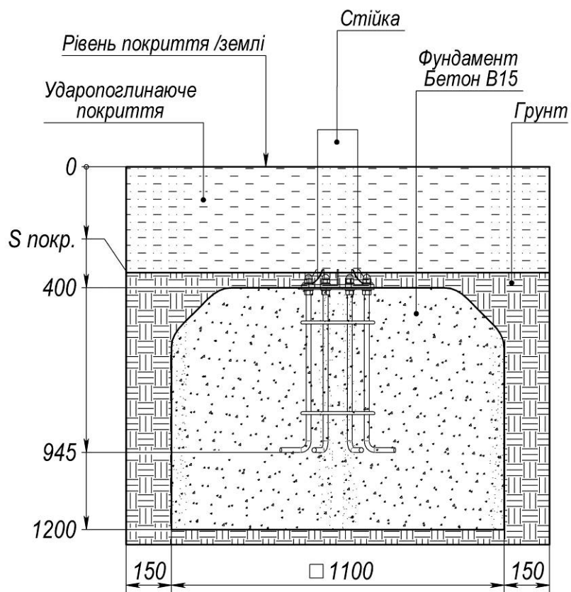
Рисунок 1 - Схема бетонування закладної
