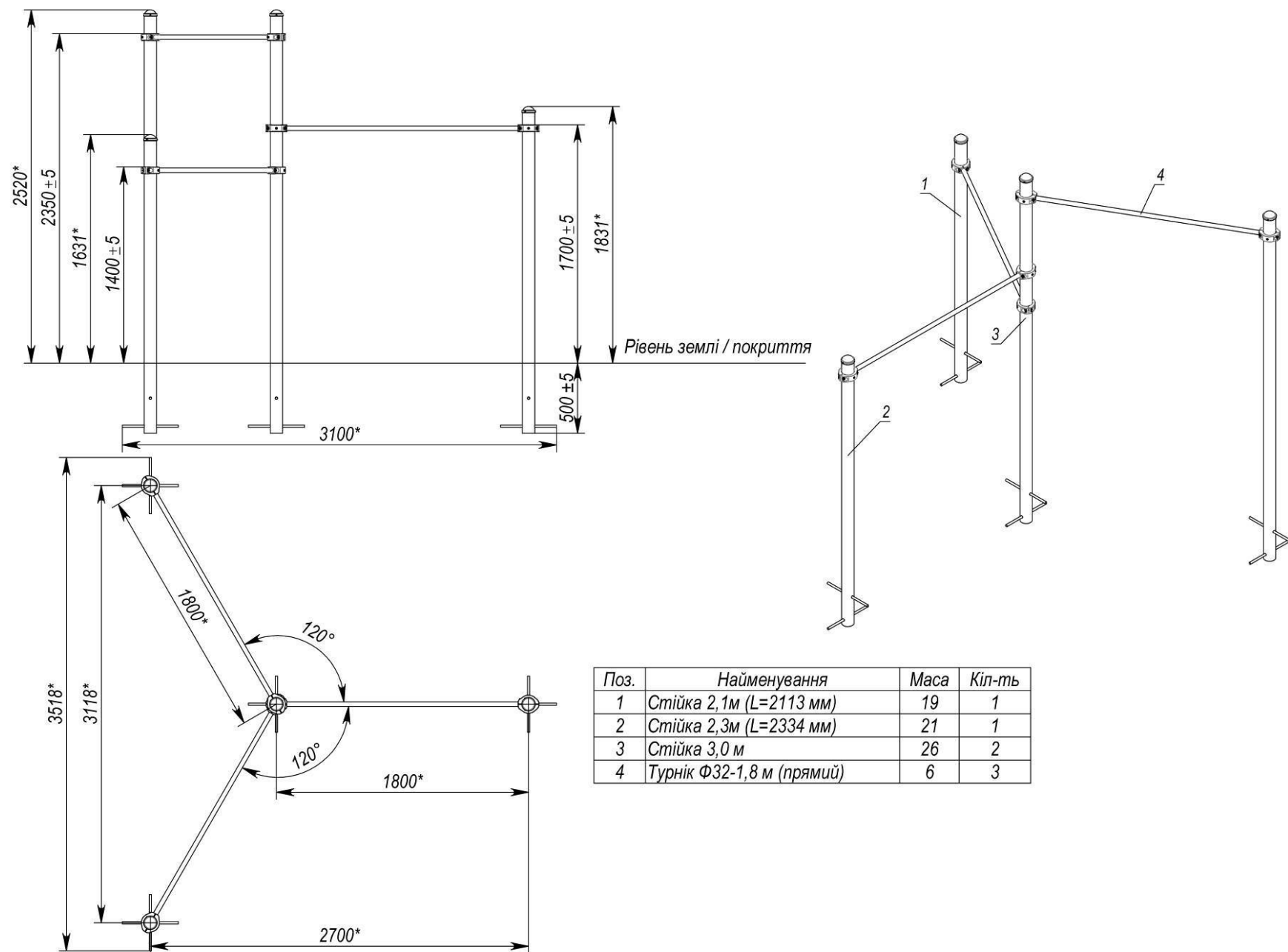
Рисунок 4 – для S832.6-UA Сторінка 26
