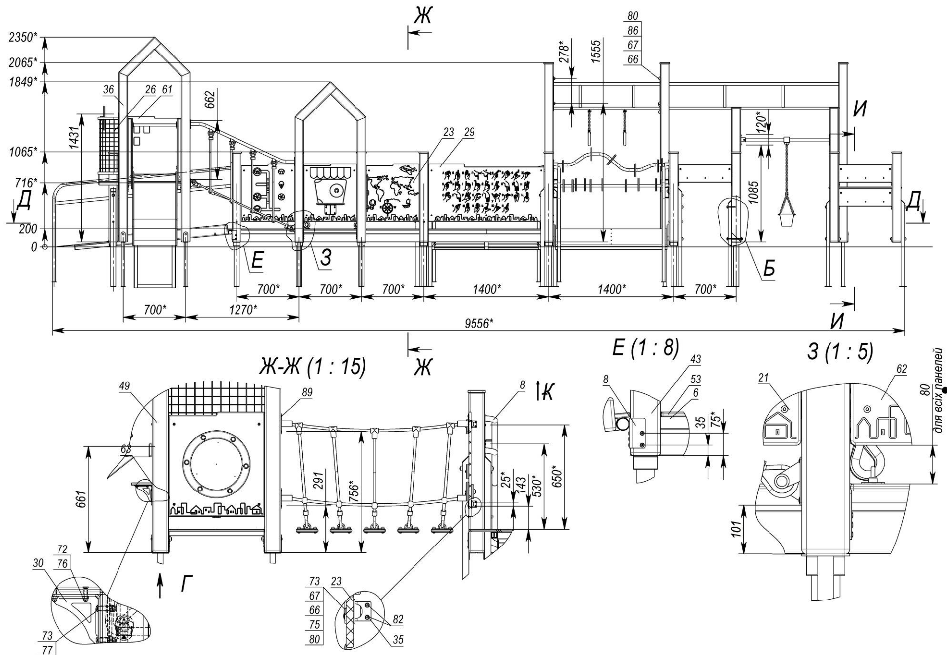
Рисунок 3 - Габаритні розміри комплексу
