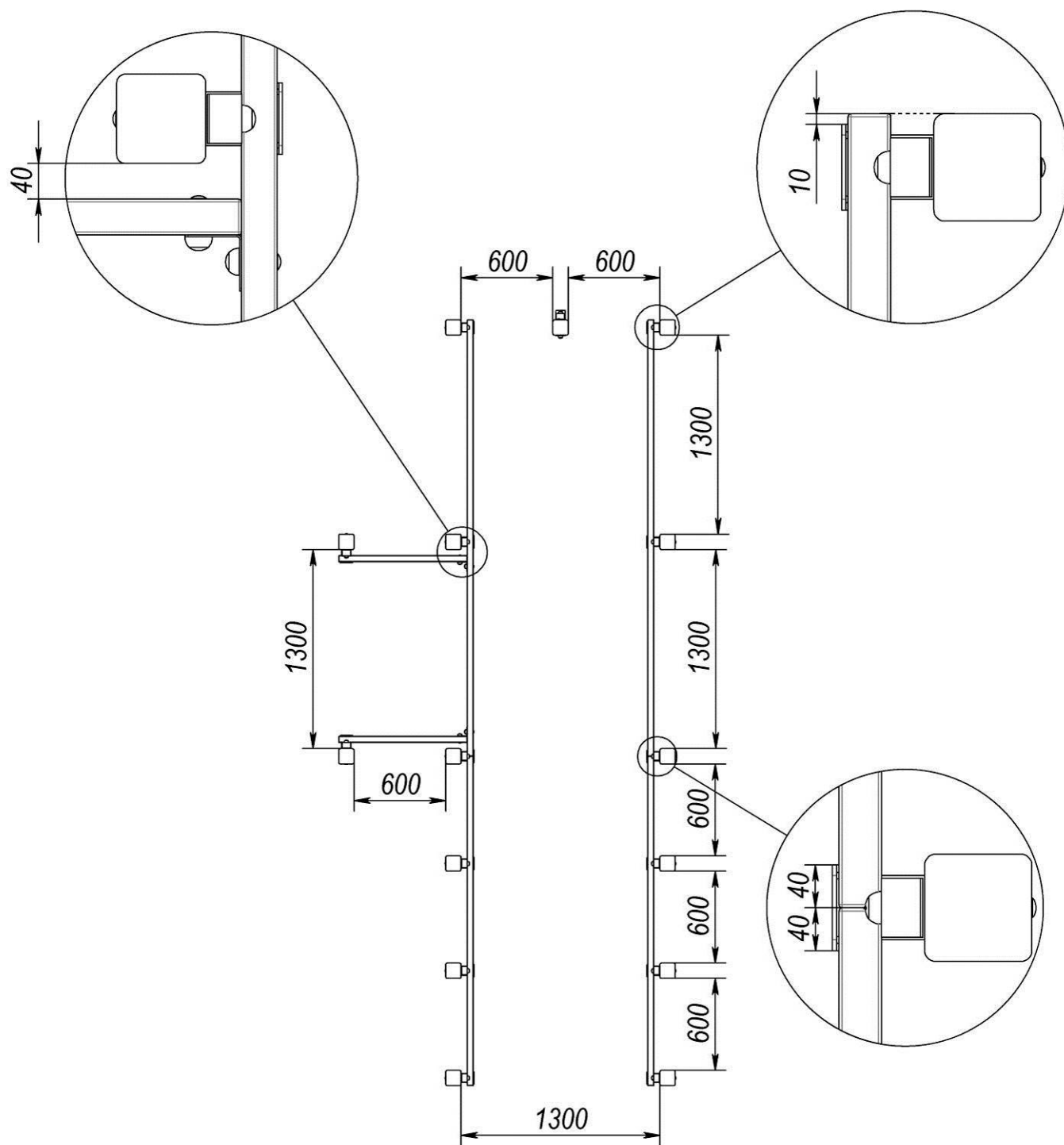
Рисунок 6 – Додатково до (схем складання опор та дошок)
