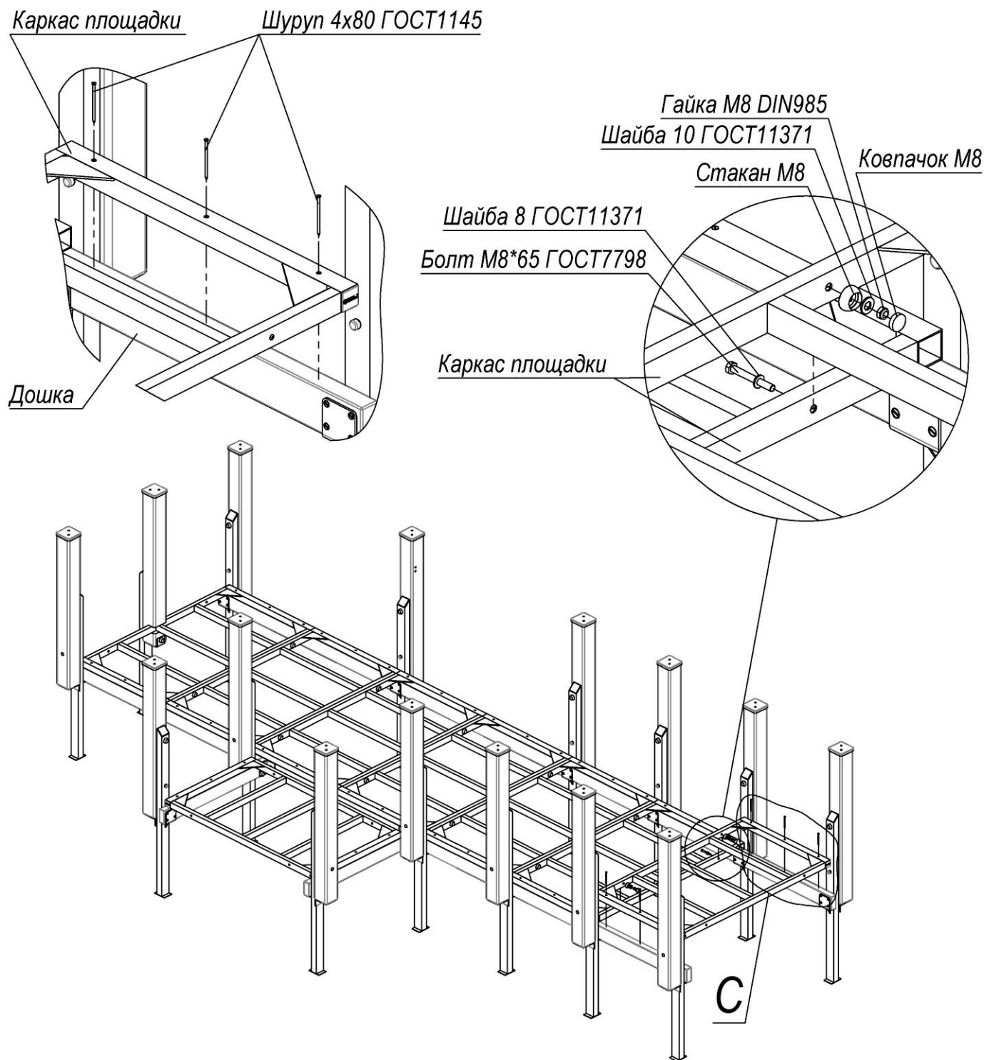
Рисунок 7 – Схема монтажу каркасу площадки
