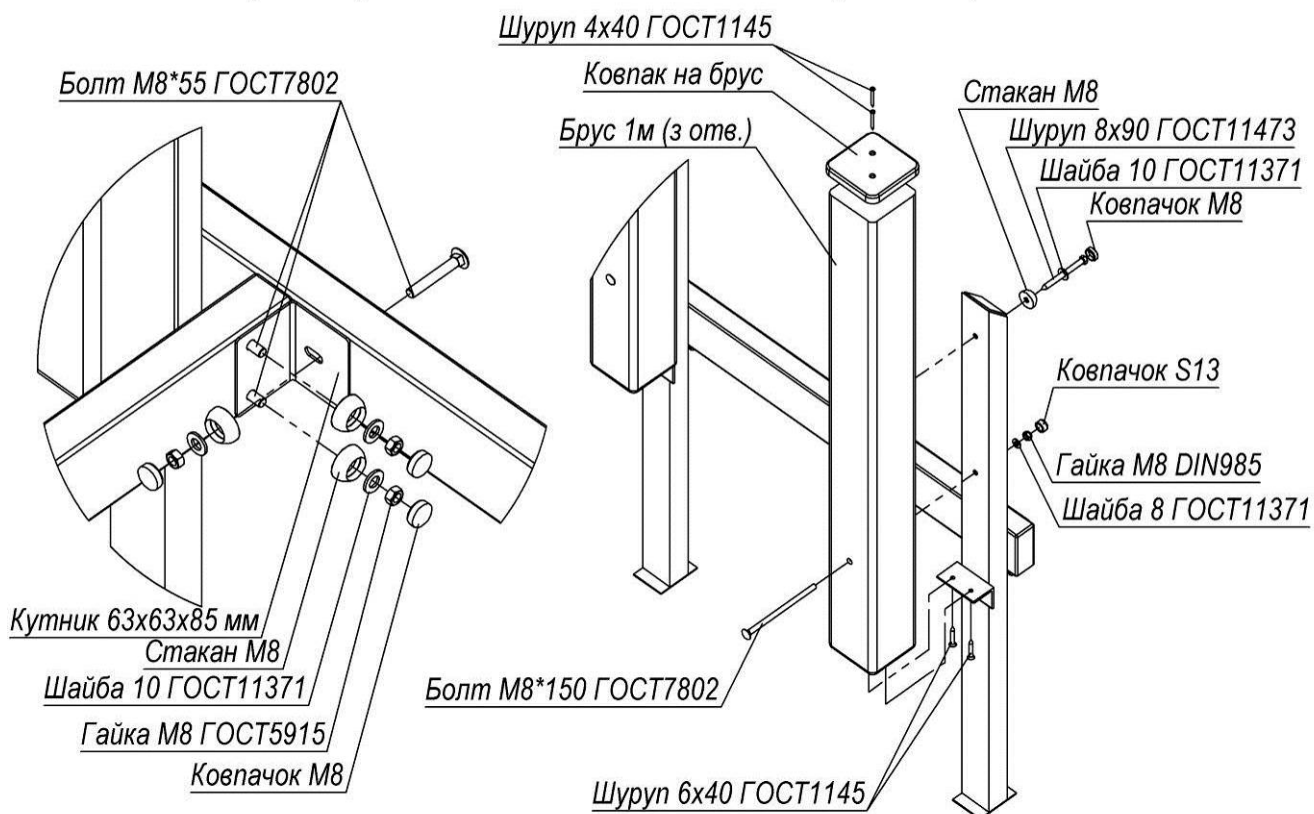
Рисунок 5 - Схема складання опор та дошок
