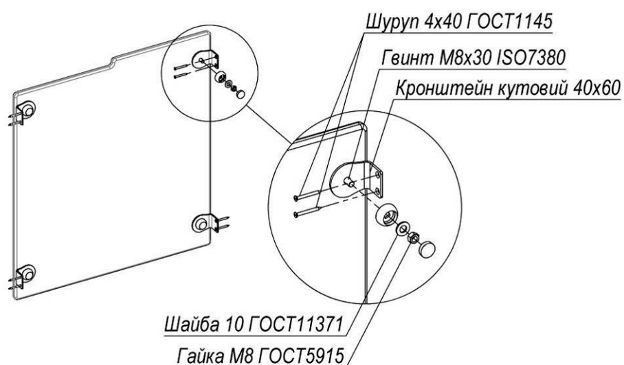
Рисунок 12 – Схема закріплення панелей
