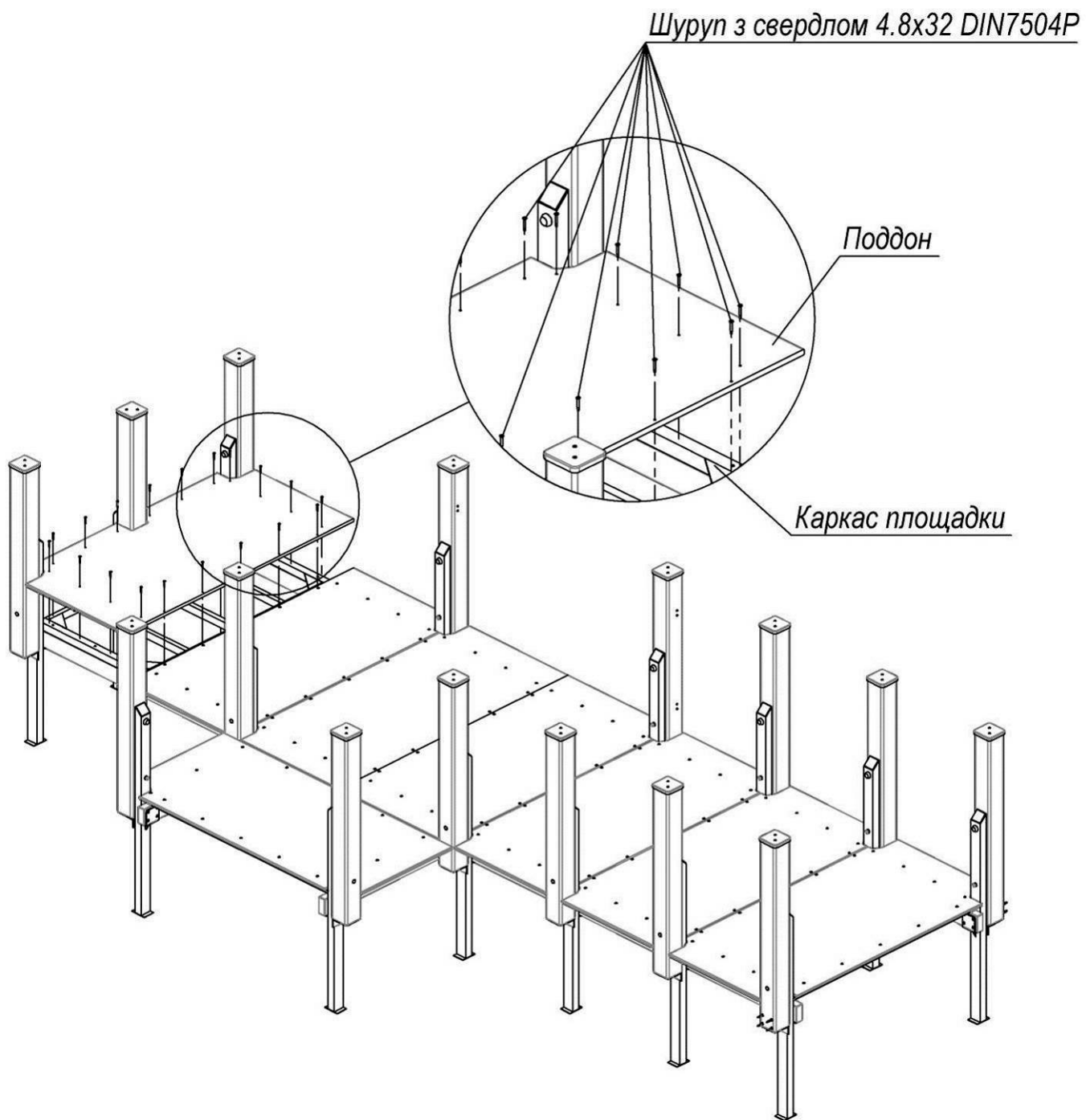
Рисунок 10 – Встановлення та закріплення піддонів
