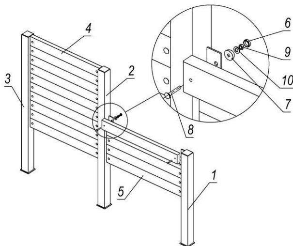
Таблиця 3 – Схема складання
