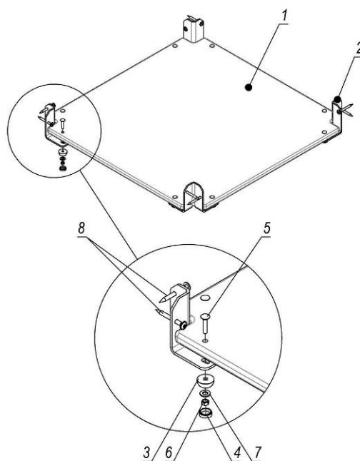
Рисунок 6 – Схема складання стійки 2м
