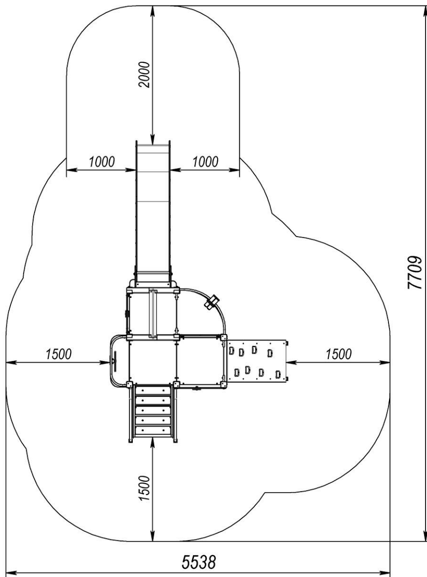
Рисунок 1 -Площа для монтажу та зона приземлення
