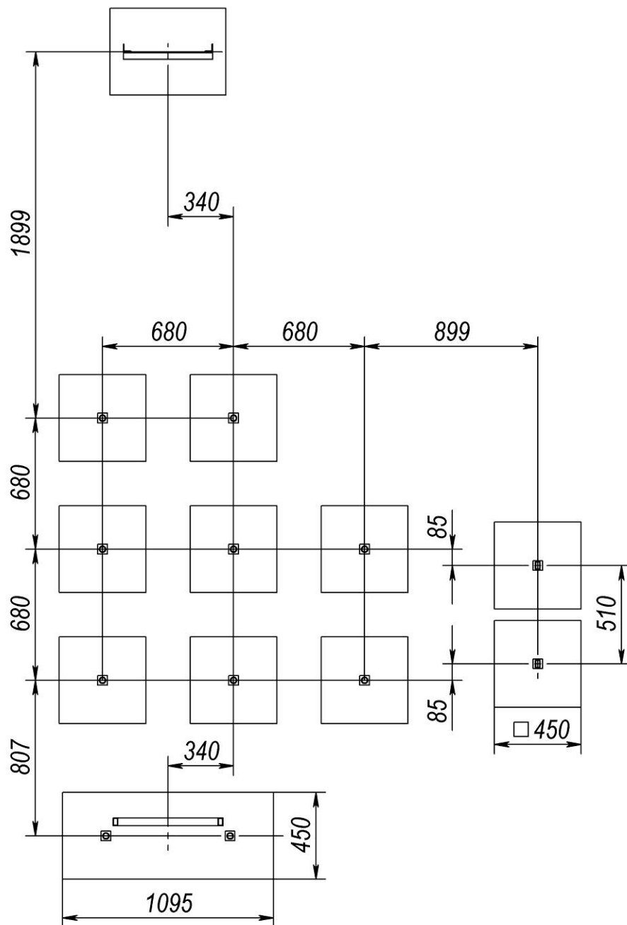
Рисунок 2 – Схема розташування фундаментів
