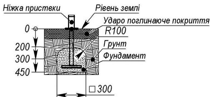
Рисунок 1 – Схеми бетонування
