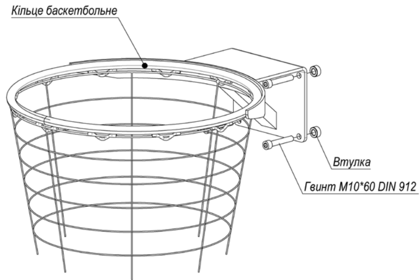
Рисунок 3 – Кріплення кільця баскетбольного під щит акриловий (для УТ409.1-01)
