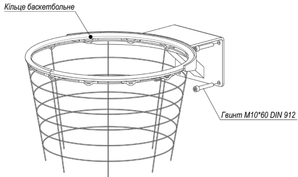
Рисунок 3 – Кріплення кільця баскетбольного під щит акриловий (для УТ409.1-01)
