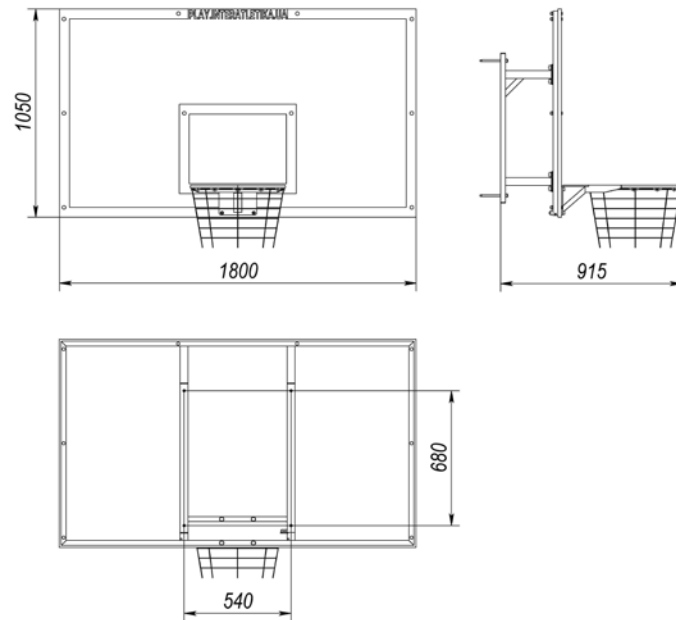
Рисунок 1 – Габаритні розміри
