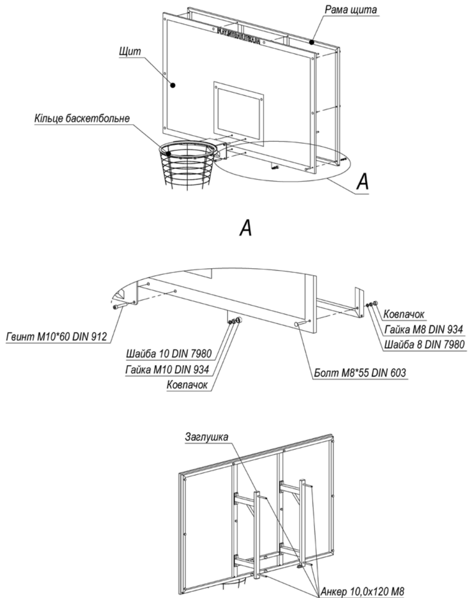
Рисунок 2 – Схема складання
