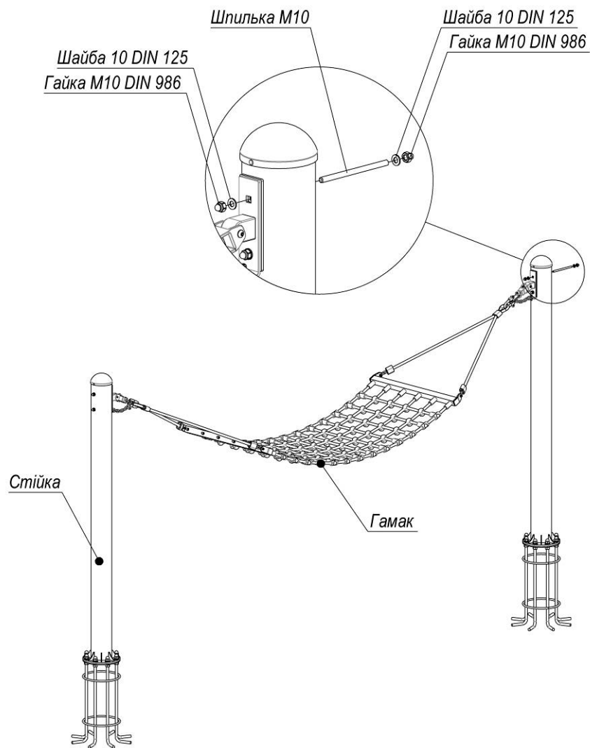
Рисунок 1 – Схема складання «Гамака»
