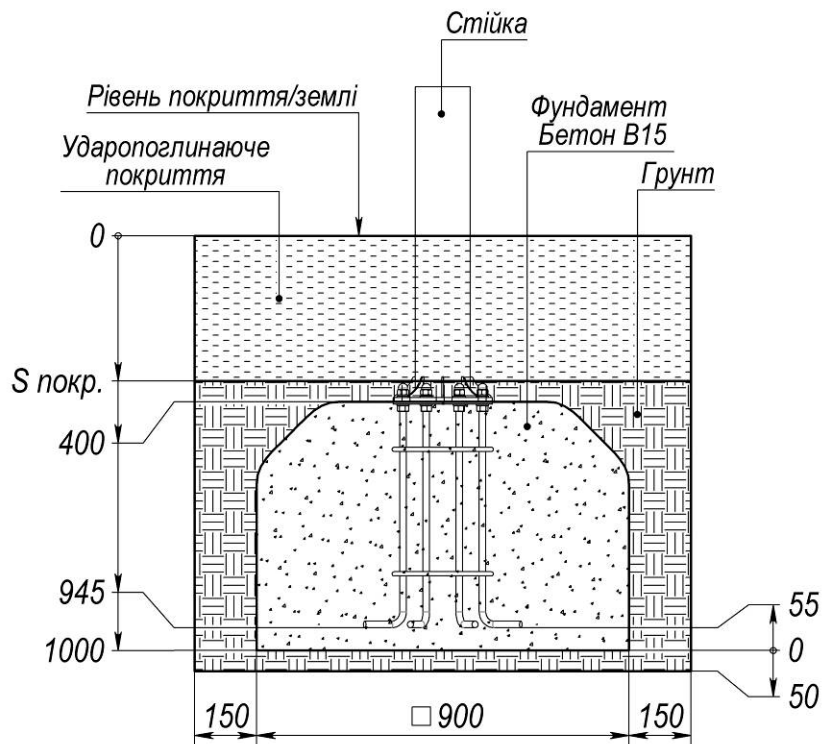
Рисунок 2 - Схема бетонування
