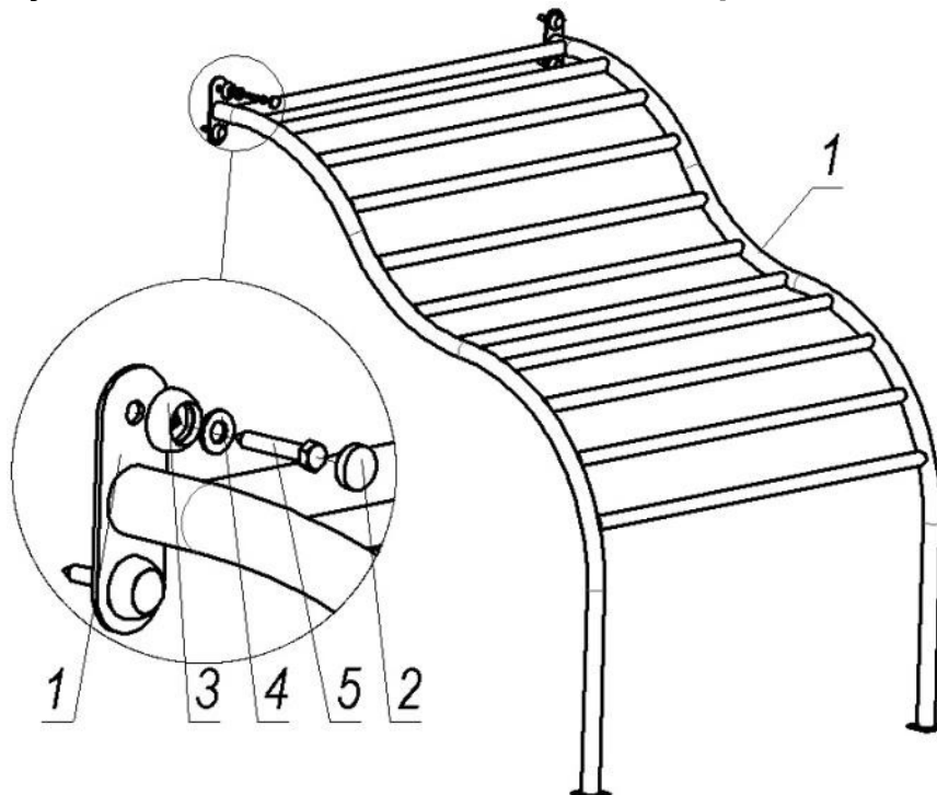
Рисунок 8 - Комплектність та схема складання ступінчатих сходів
