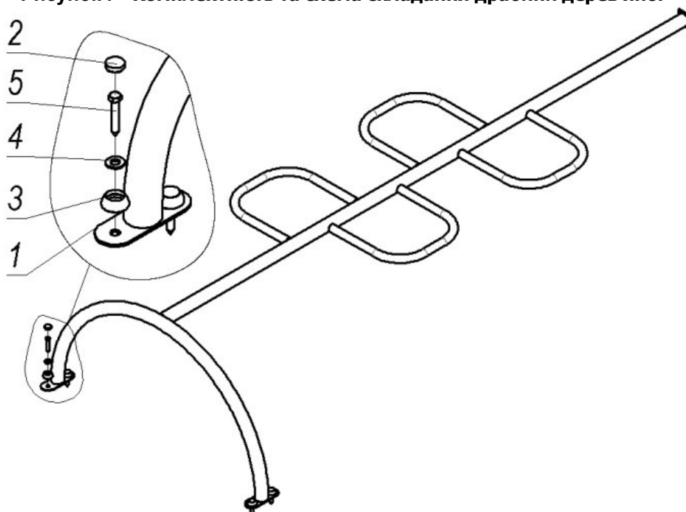
Рисунок 7 - Комплектність та схема складання драбини дерев'яної
