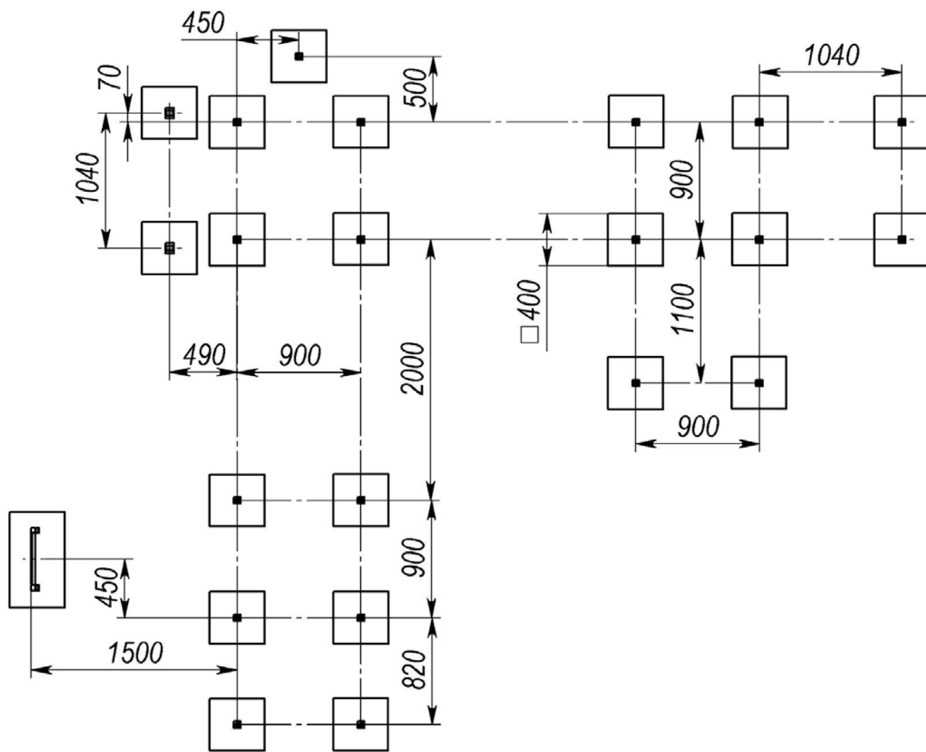
Рисунок 17 - Схема розташування фундаментів
