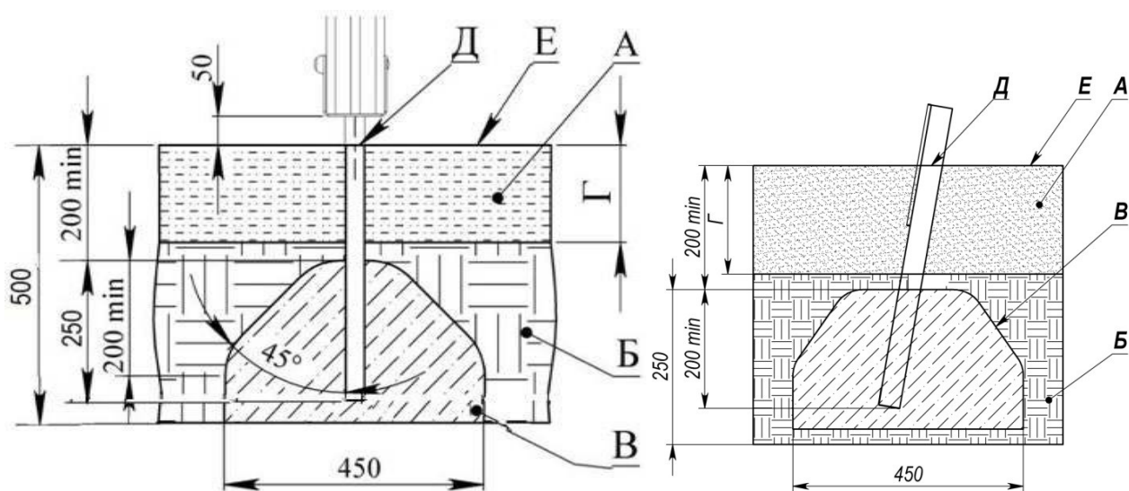
Рисунок 17 - Схема розташування фундаментів
