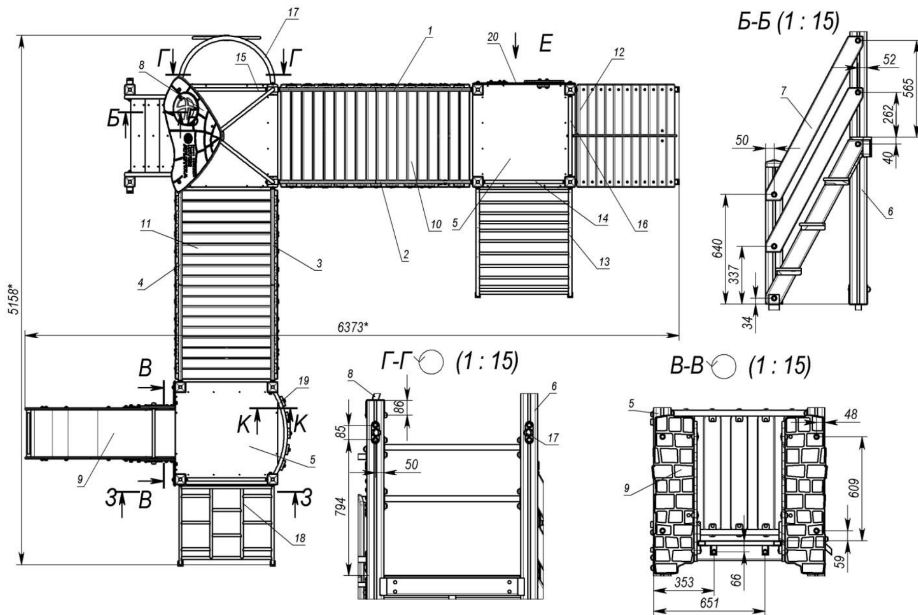
Рисунок 1 - Комплектація та характеристики складових частин виробу
