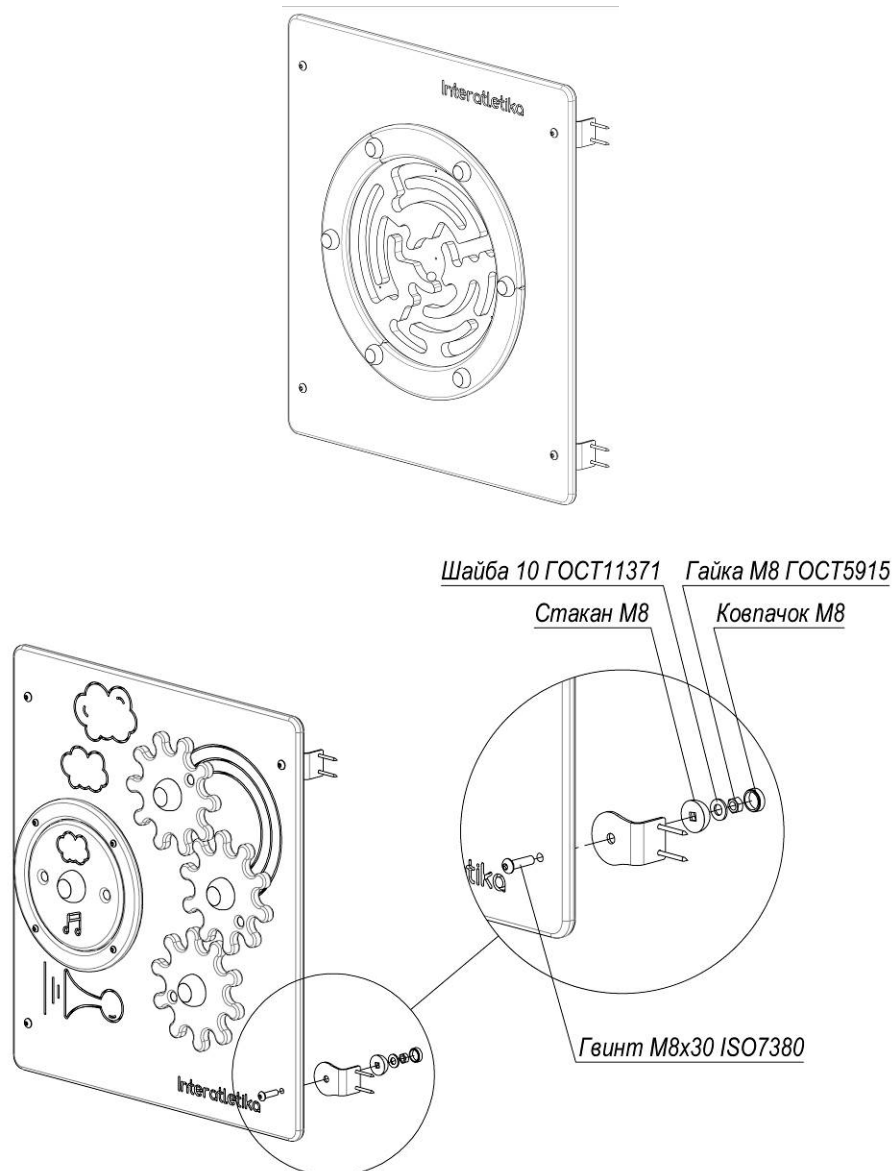
Рисунок 8 – Панель з вентилями, Лабіринт вертикальний
