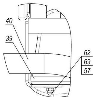
Б (1 : 2.5)
