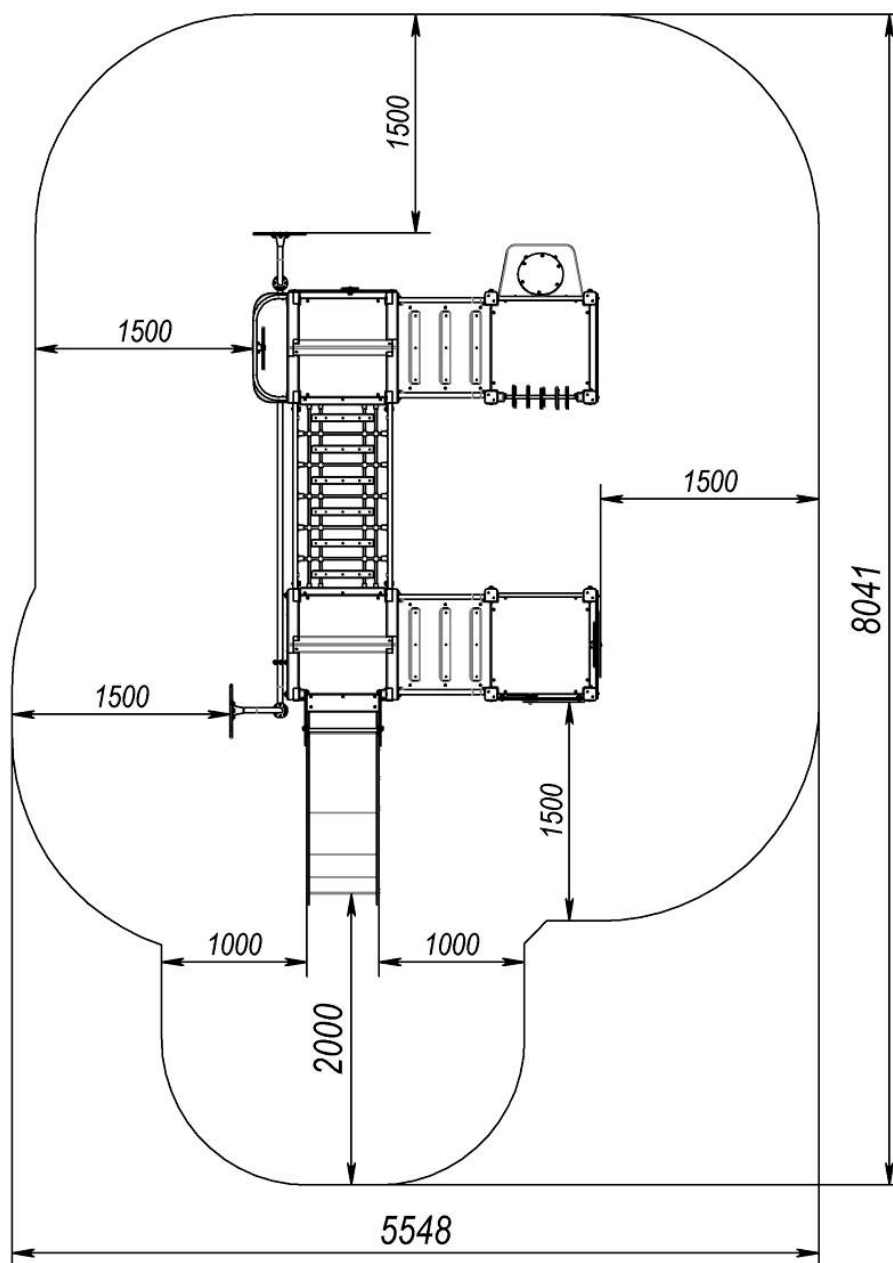
Рисунок 1 -Площа для монтажу та зона приземлення
