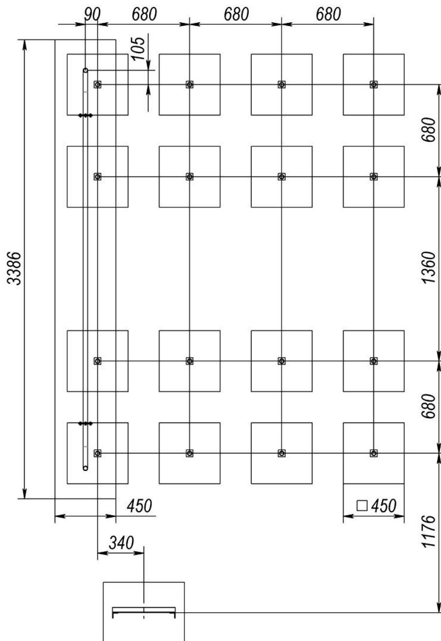
Рисунок 2 – Схема розташування фундаментів
