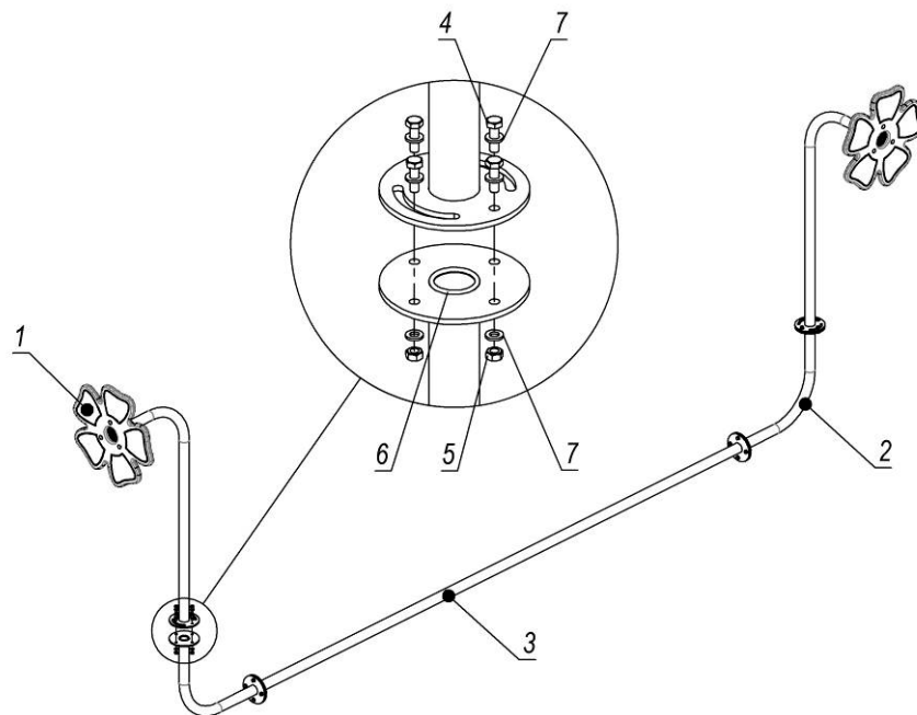
Рисунок 7 – Схема складання панелі (складання інших панелей ідентична)
