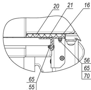
В-В (1 : 4)
