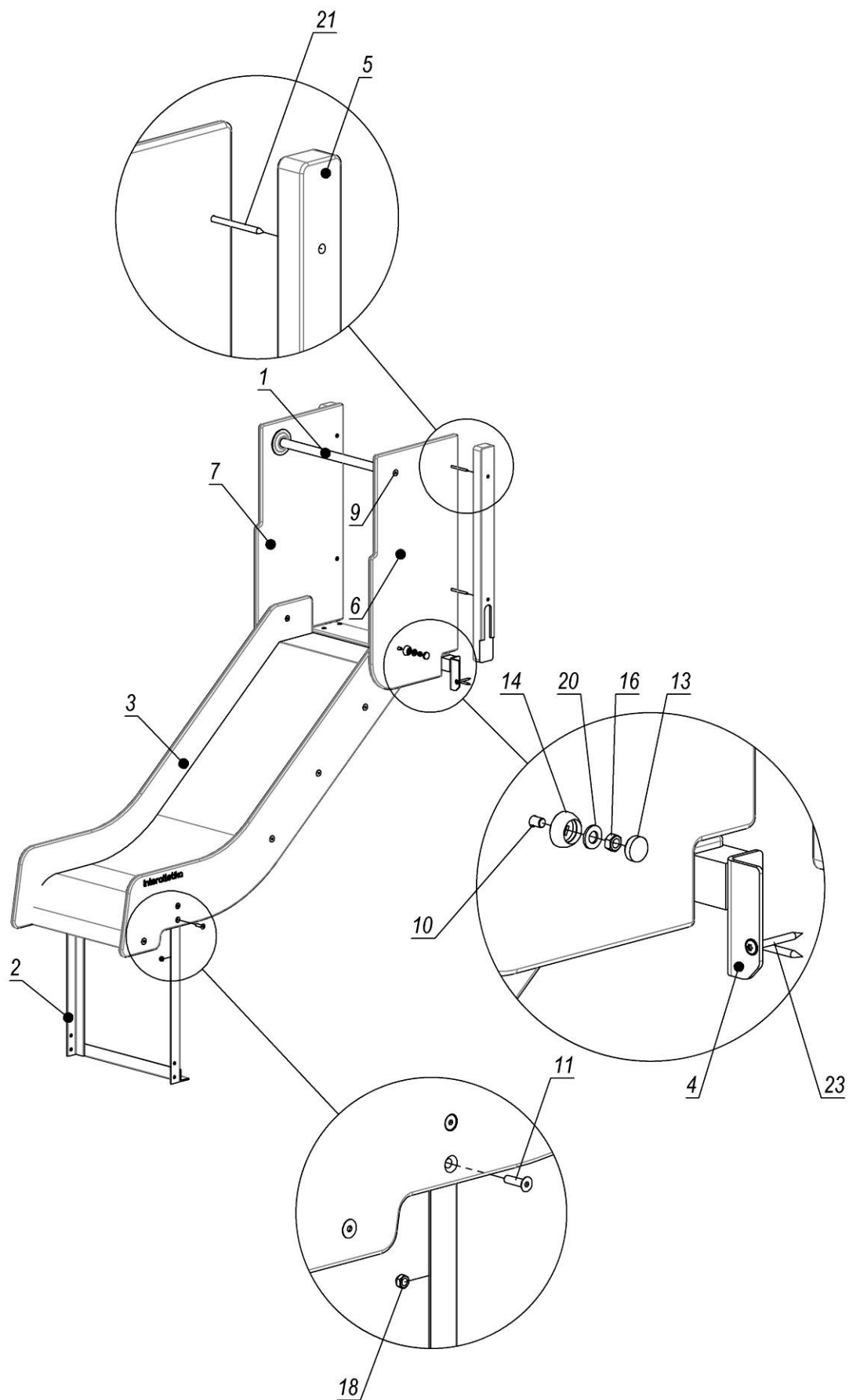
Рисунок 5 - Схема складання гірки
