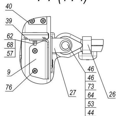
Г-Г (1 : 4)
