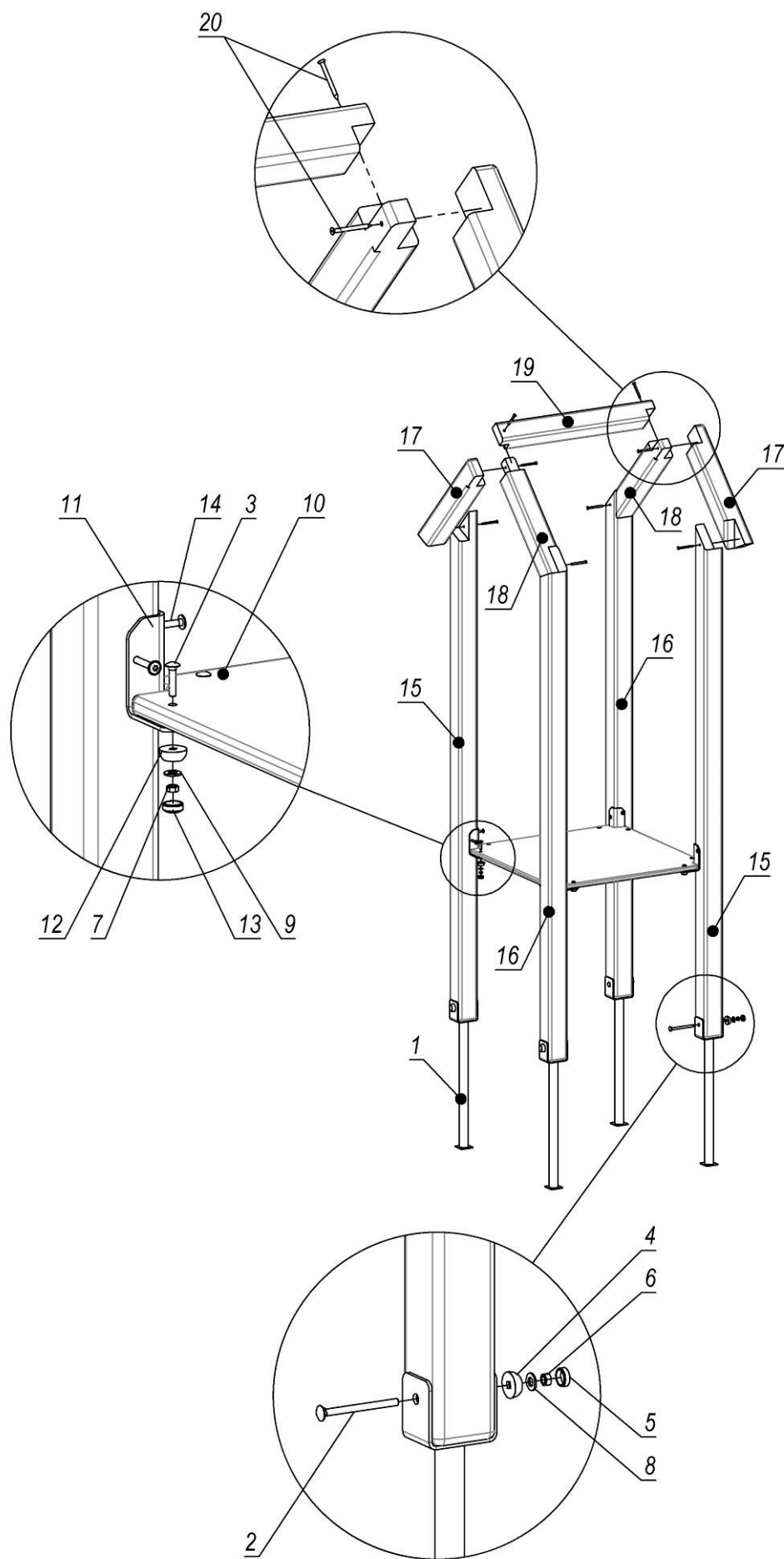
Рисунок 3 – Схема складання вежі
