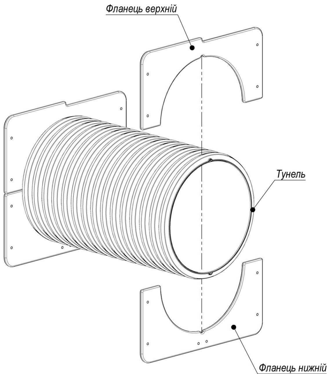
Рисунок 7 – Схема складання тунельного переходу
