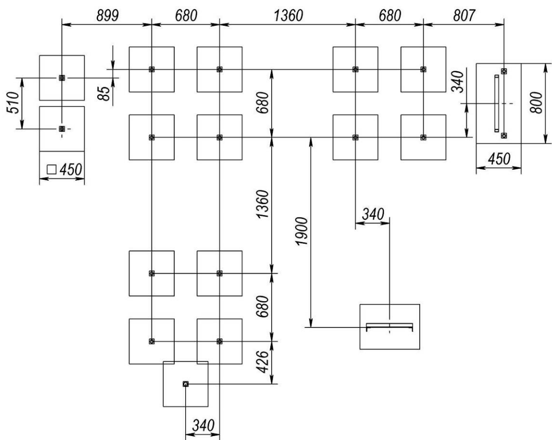
Рисунок 2 – Схема розташування фундаментів
