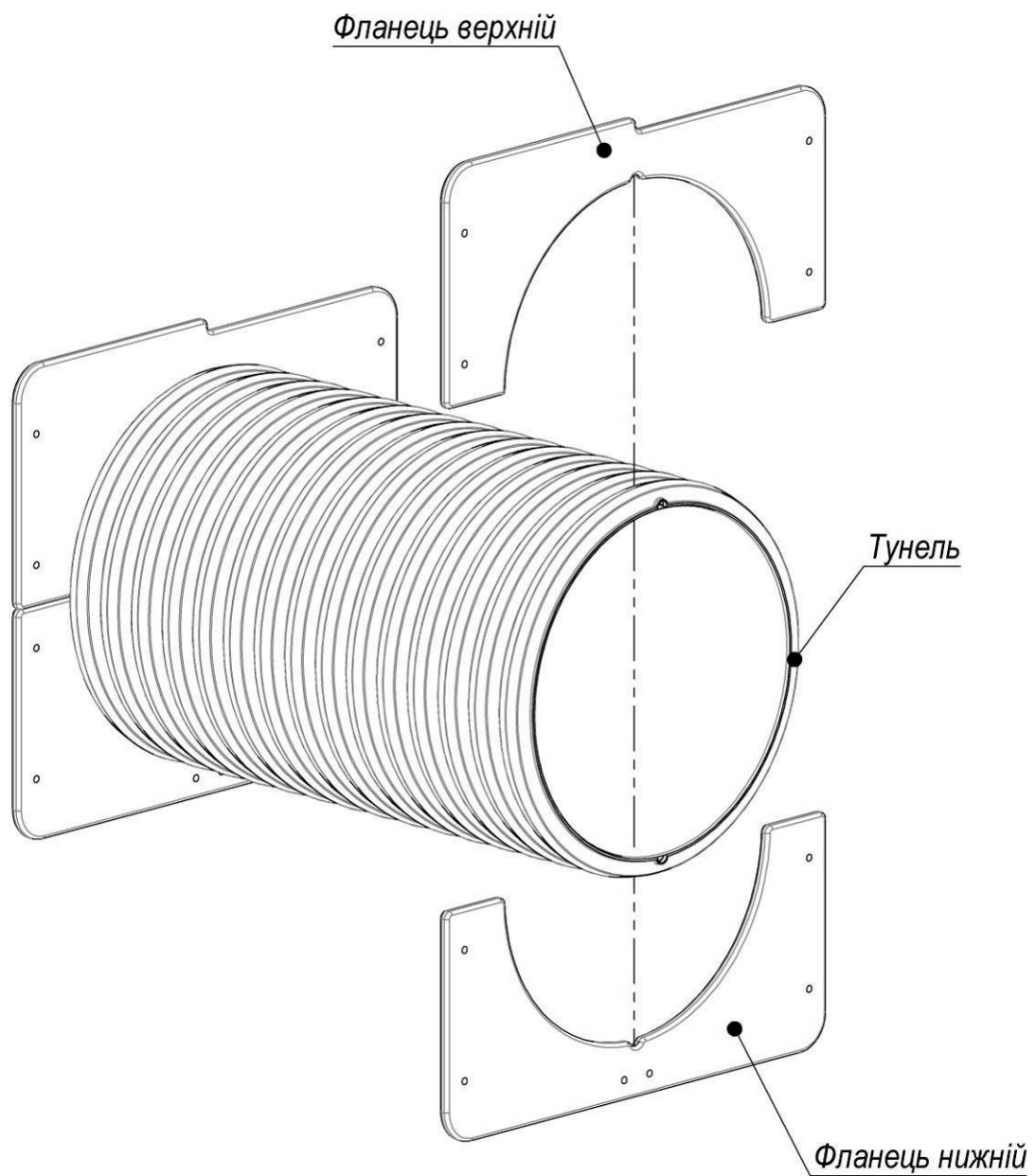
Рисунок 9 – Схема складання тунельного переходу
