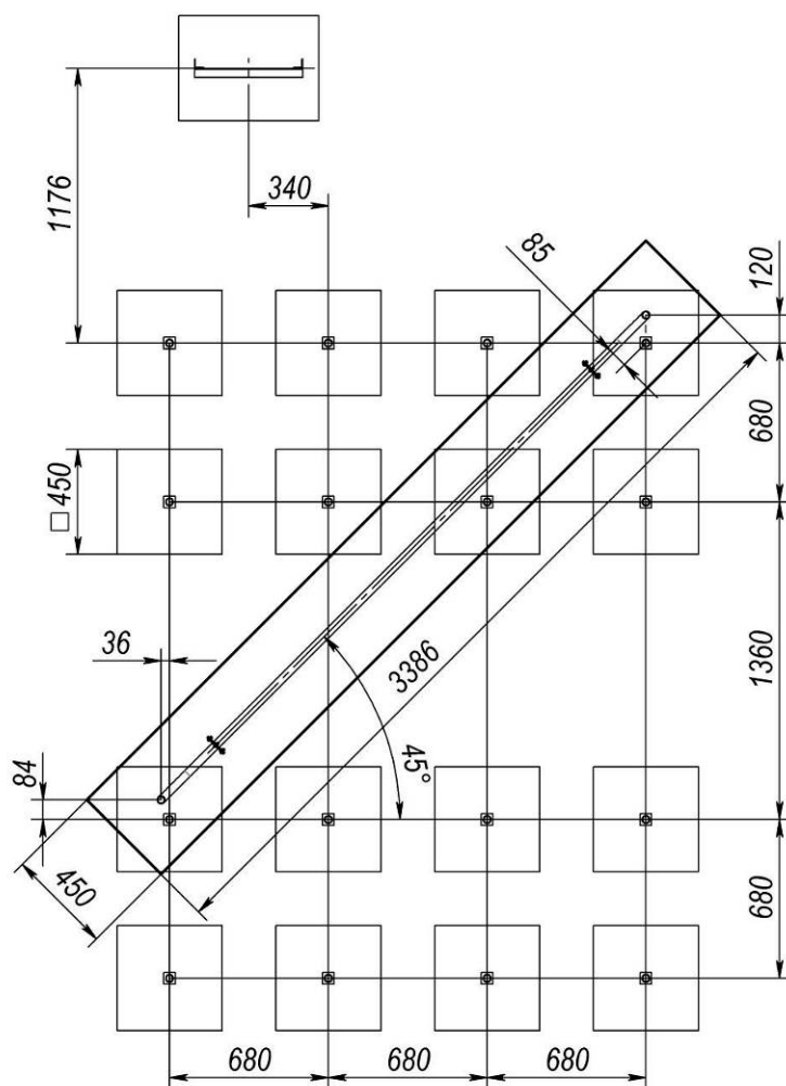
Рисунок 2 – Схема розташування фундаментів
