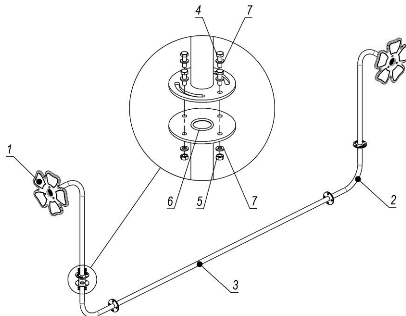
Рисунок 6 – Схема складання панелі (складання інших панелей ідентична)
