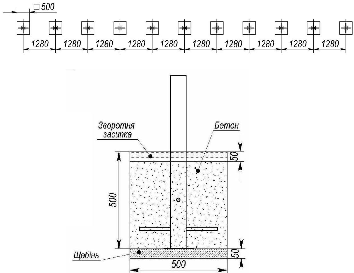
Рисунок 3 – Зона бетонування
