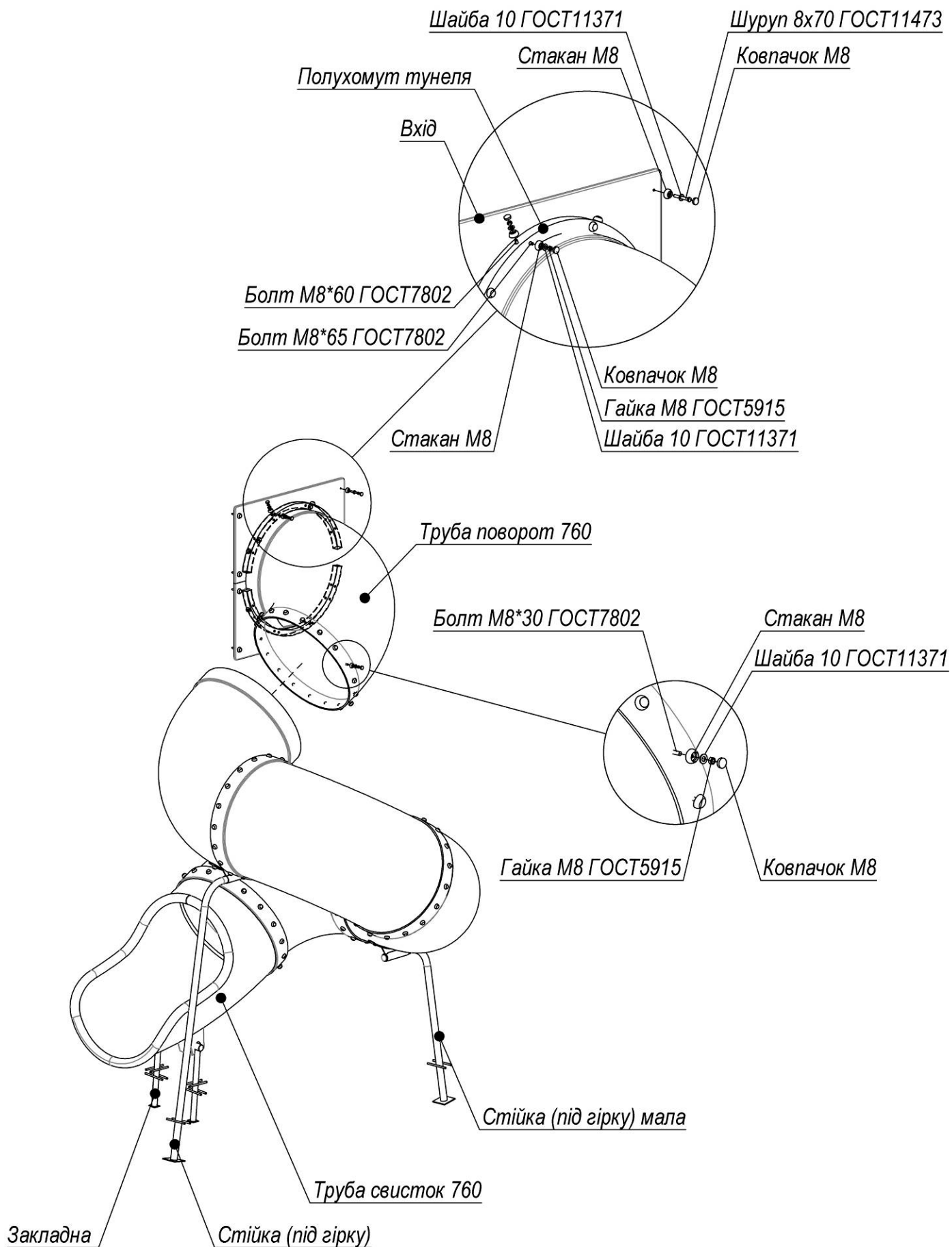
Рисунок 14 – Схема збирання гірки Укрхімпласт. (Додатково схема збирання в додатку)
