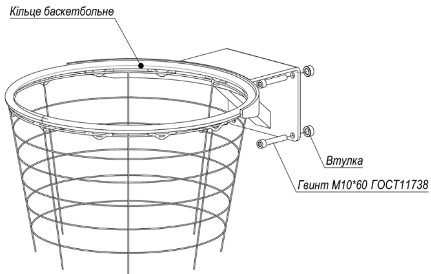
Рисунок 4 – Кріплення кільця баскетбольного під щит акриловий (для УТ406.1-01)
