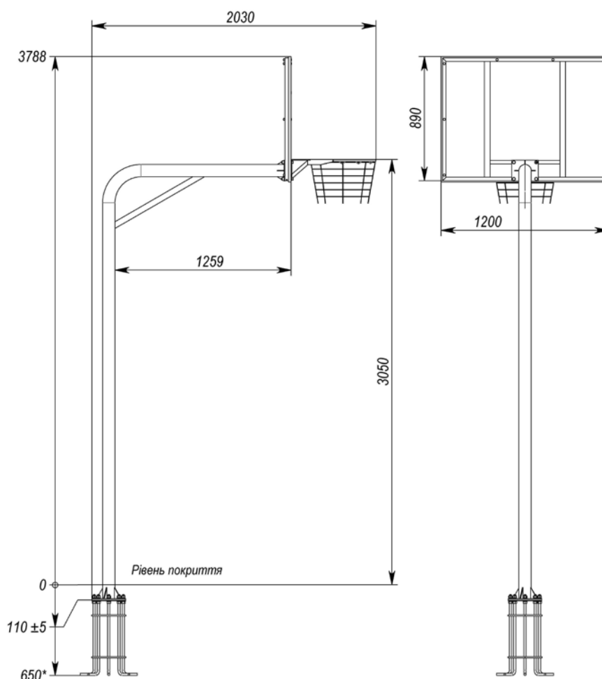
Рисунок 1 – Габаритні розміри
