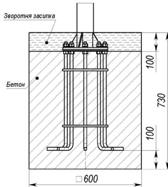
Рисунок 3 – Схема бетонування
