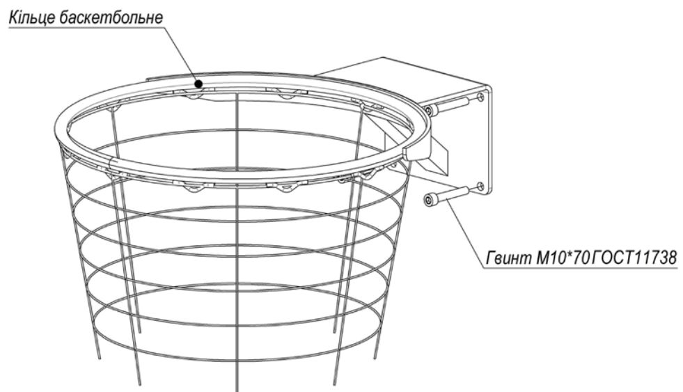
Рисунок 5 – Кріплення кільця баскетбольного під щит фанерний (для УТ406-01)
