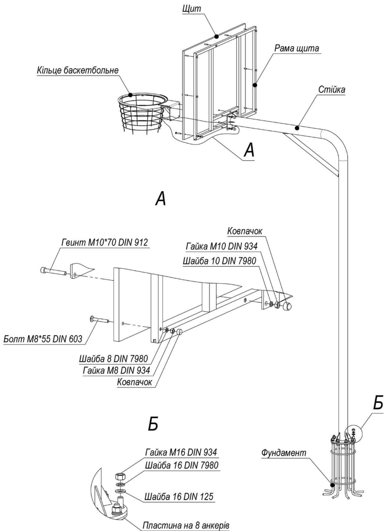
Рисунок 2 – Схема складання
