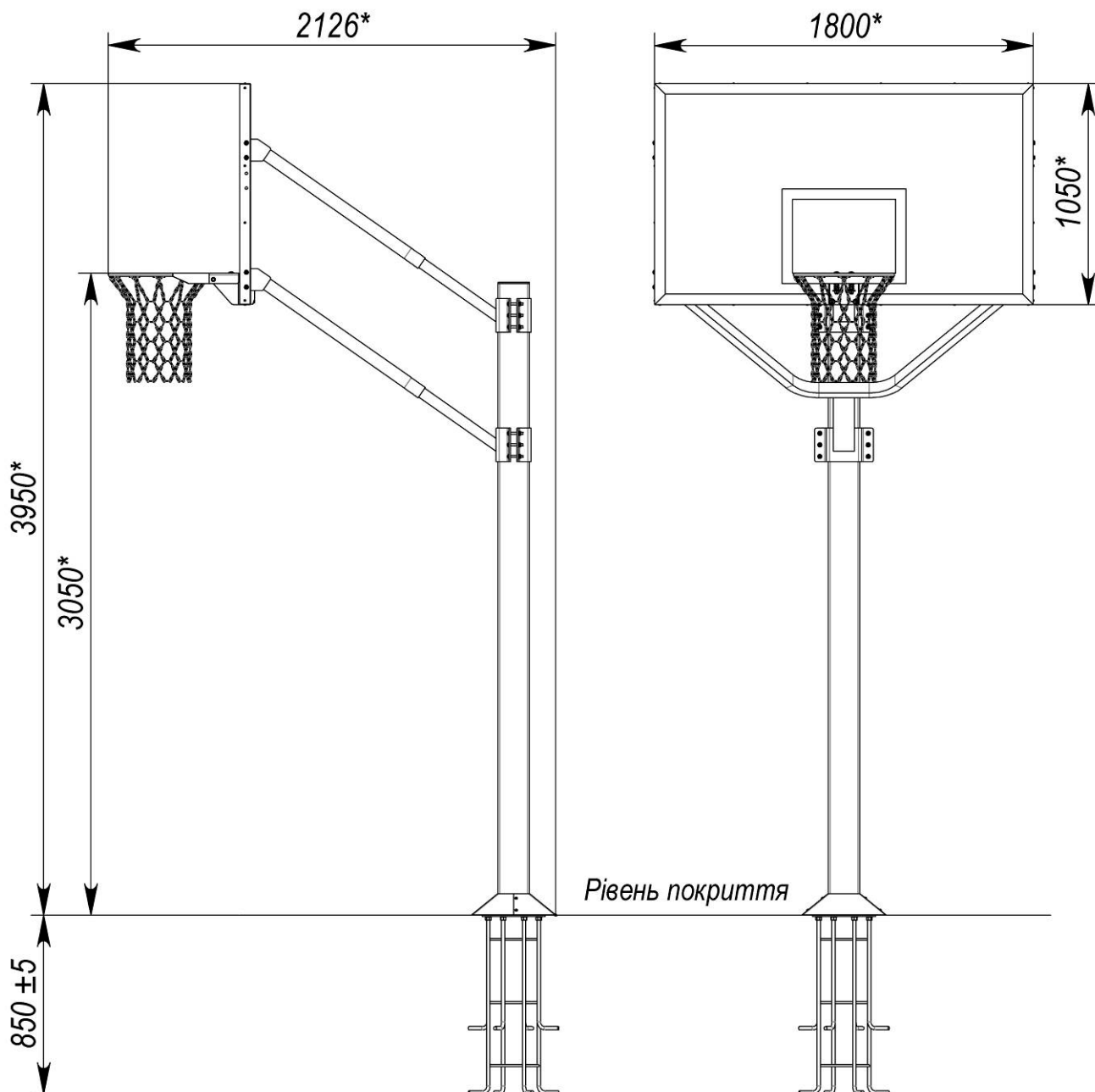
Рисунок 1 – Габаритні розміри
