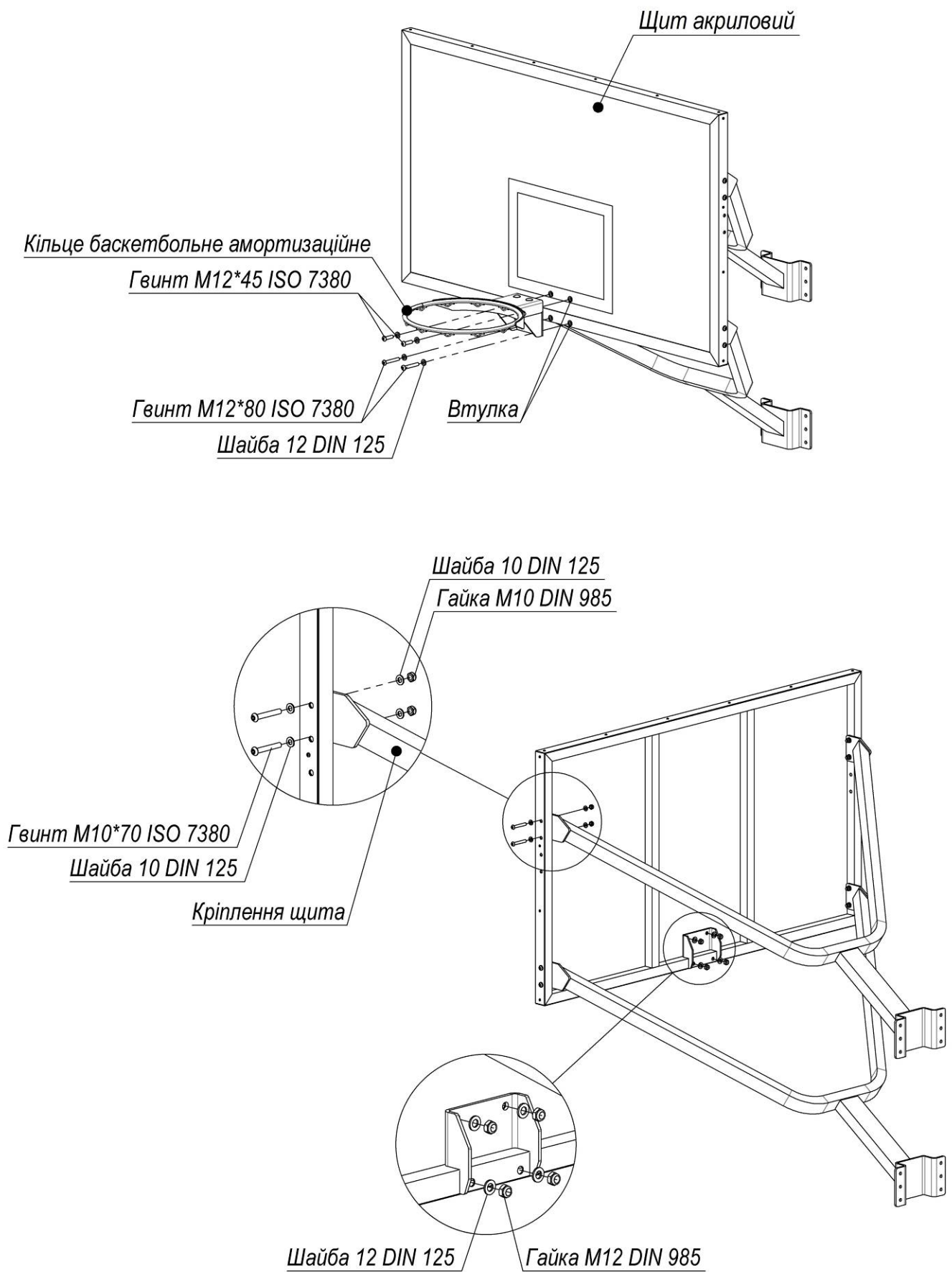
Рисунок 2 – Схема монтажу 1
