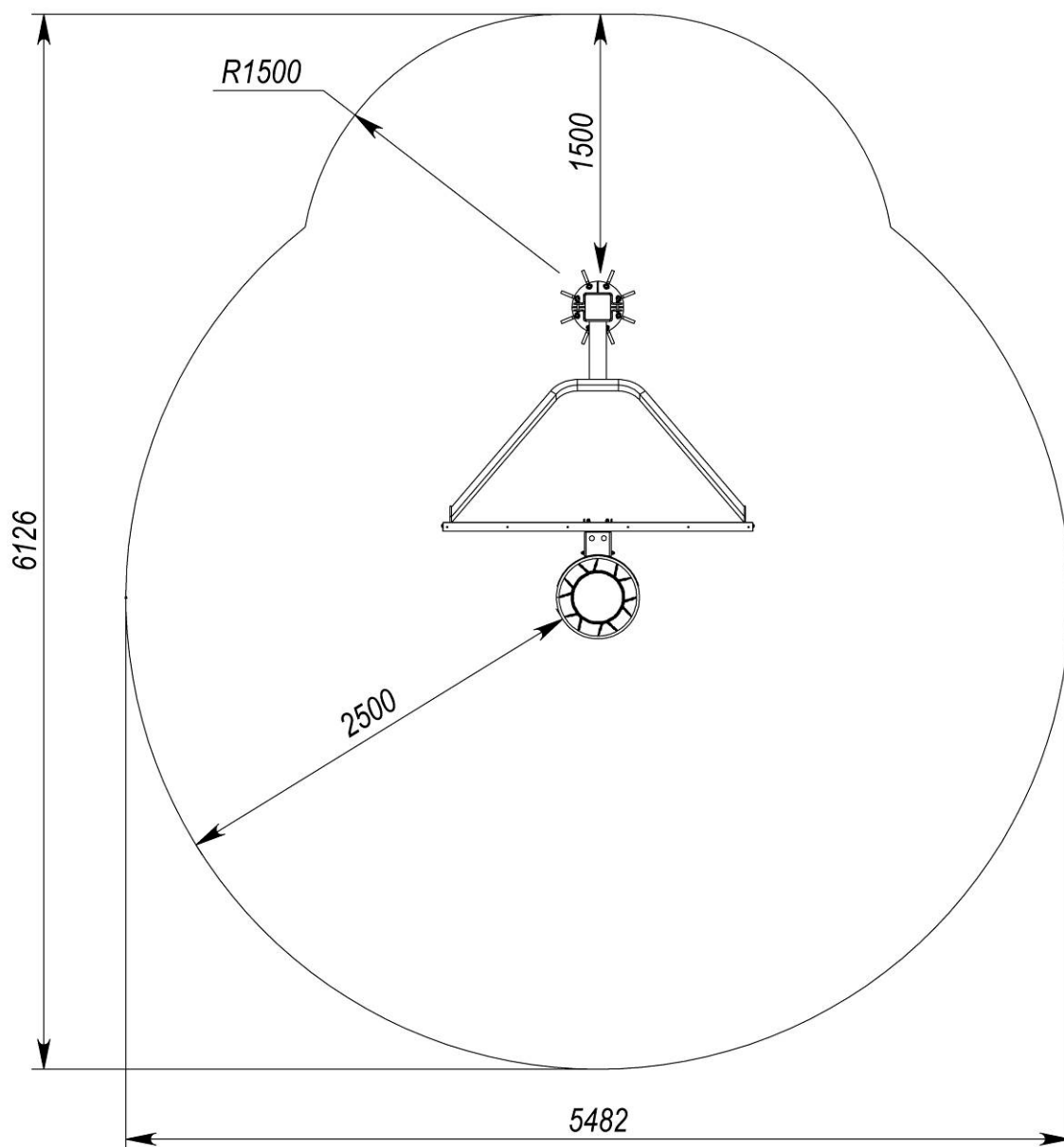
Рисунок 5 – Зона безпеки
