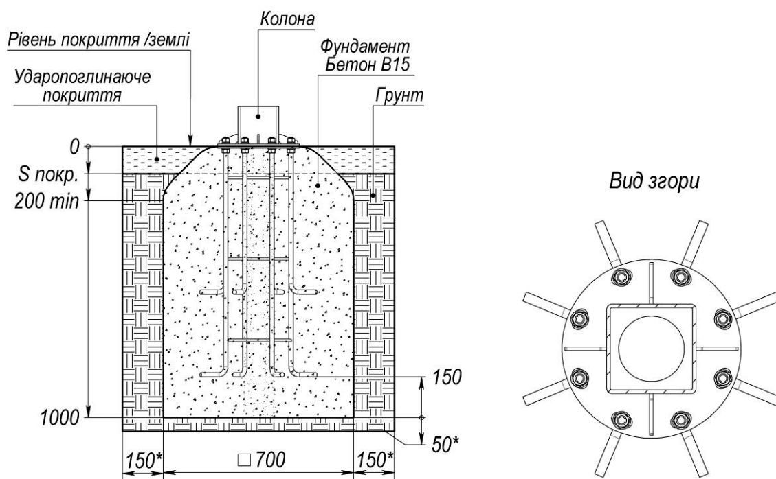
Рисунок 4 – Схема Бетонування
