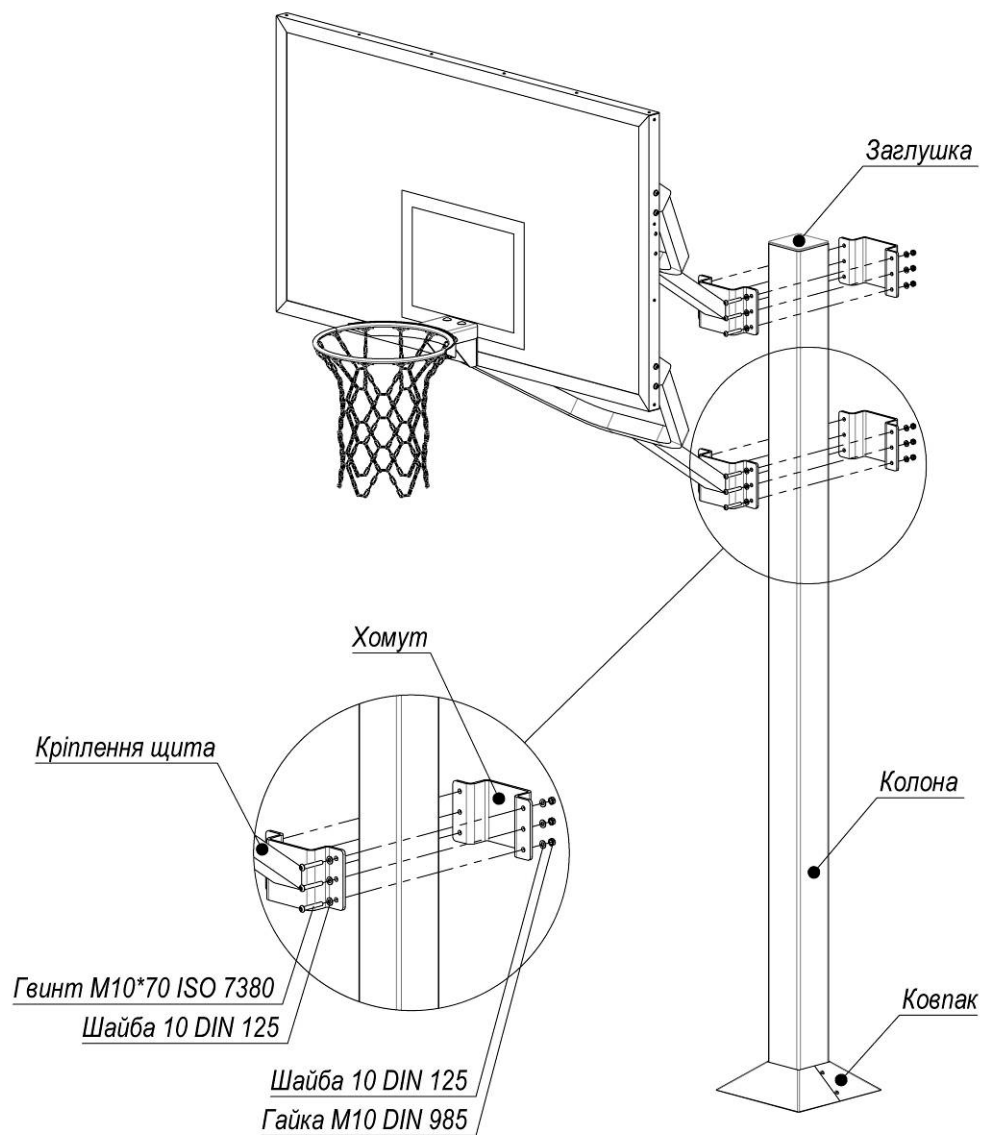
Рисунок 3 – Схема монтажу 2
