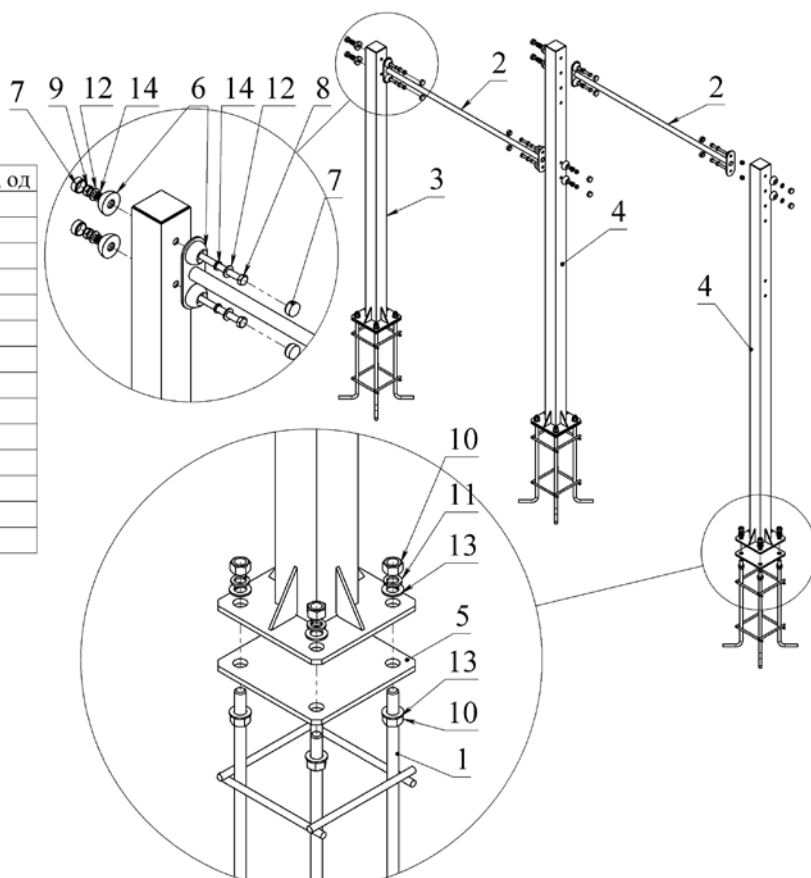
Рис. 2 Схема збирання
