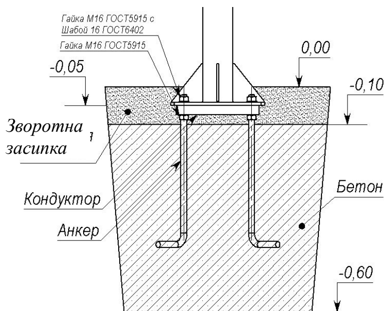
Рис. 1 Схема монтажу фундаментів
