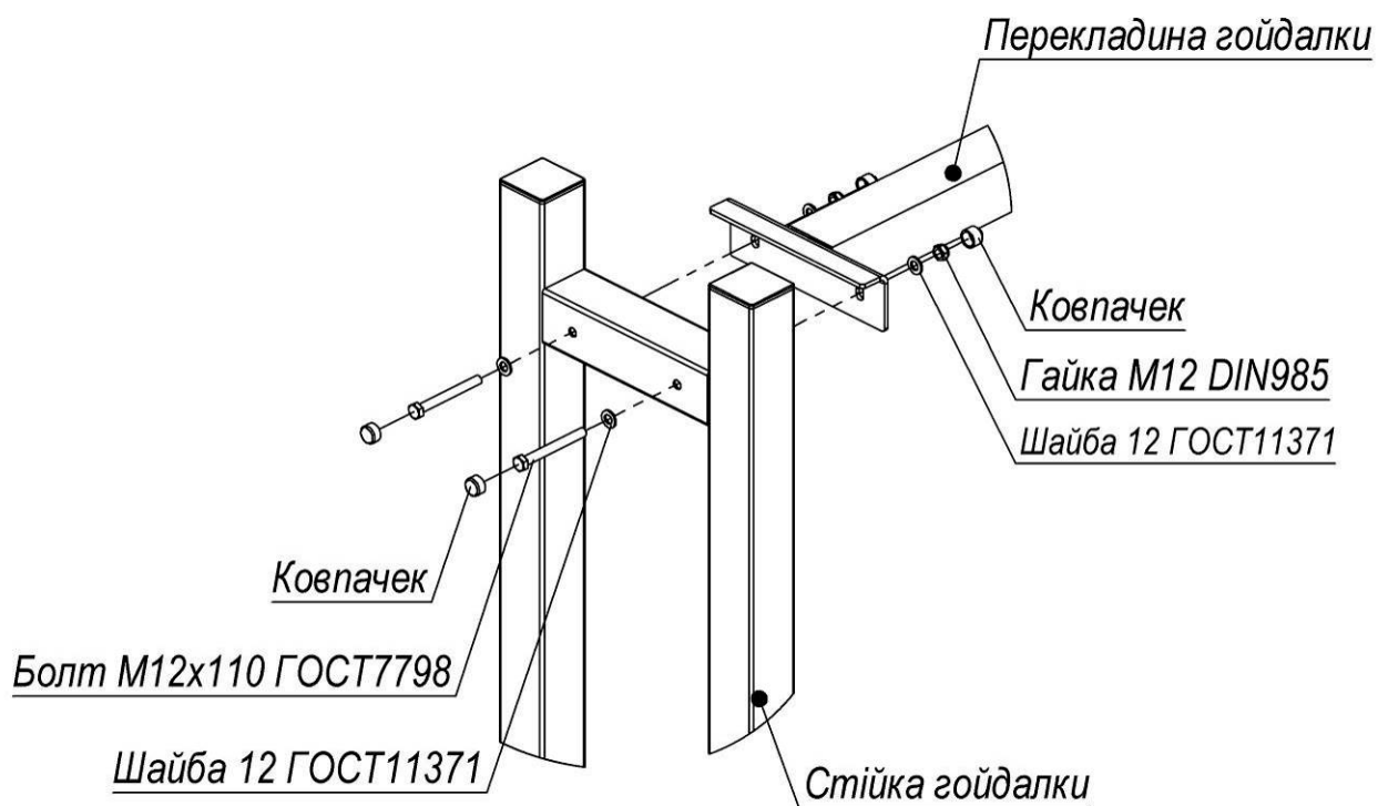
Рисунок 1 – Схема встановлення перекладини
