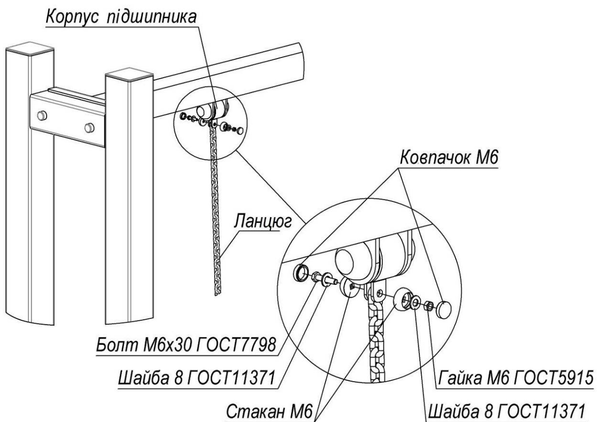
Рисунок 1 – Схема встановлення перекладини
