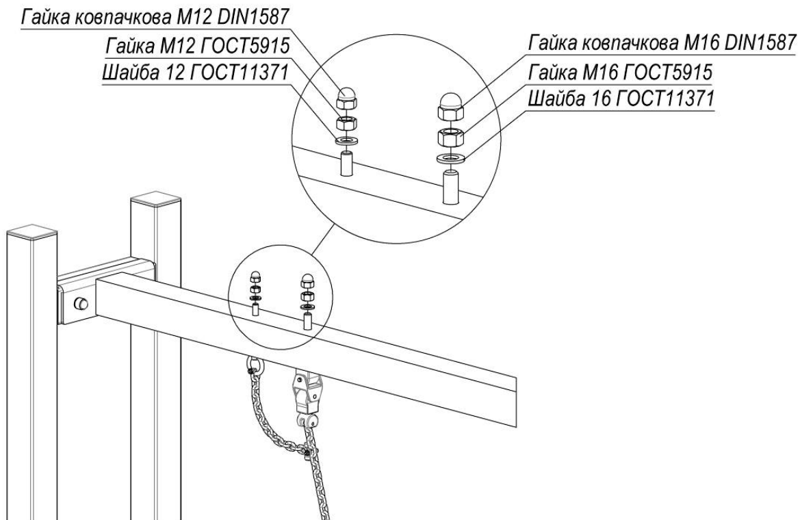
Рисунок 3 - Схема закріплення гнізда «Лелеки» для TE431-A-KBT
