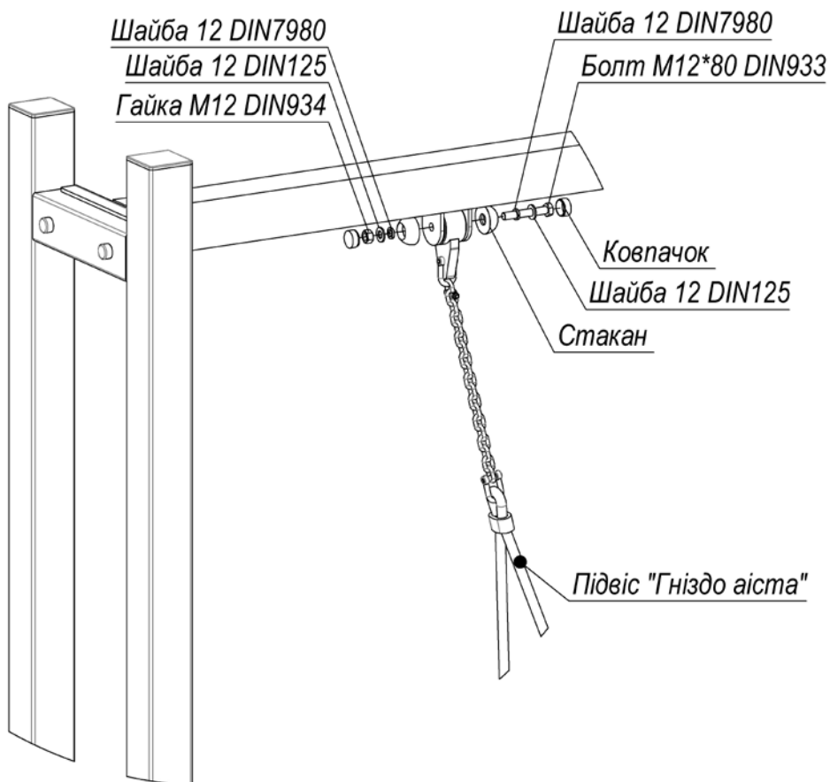
Рисунок 4 - Схема закріплення гнізда «Лелеки» для TE431-A
